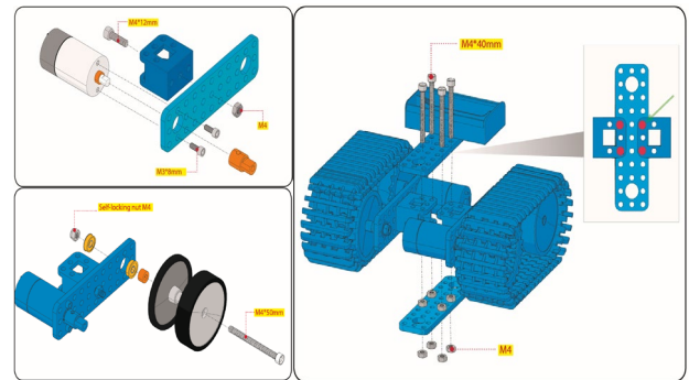
Figura 8. Ensamble del robot físico (Key Studio Tank).
