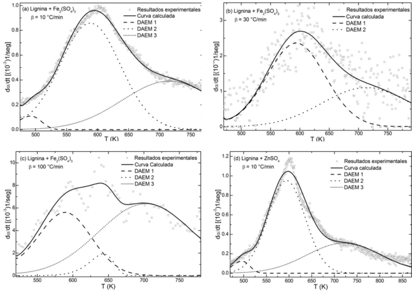
Figura 6. Ajustes de las curvas DTG de lignina con \text{Fe}_2(\text{SO}_4)_3 y lignina con \text{ZnSO}_4 a tres velocidades de calentamiento usando DAEM. Figure 6. Fit of DAEM to lignin DTG curves with \text{Fe}_2(\text{SO}_4)_3 and \text{ZnSO}_4 at three heating rates.
