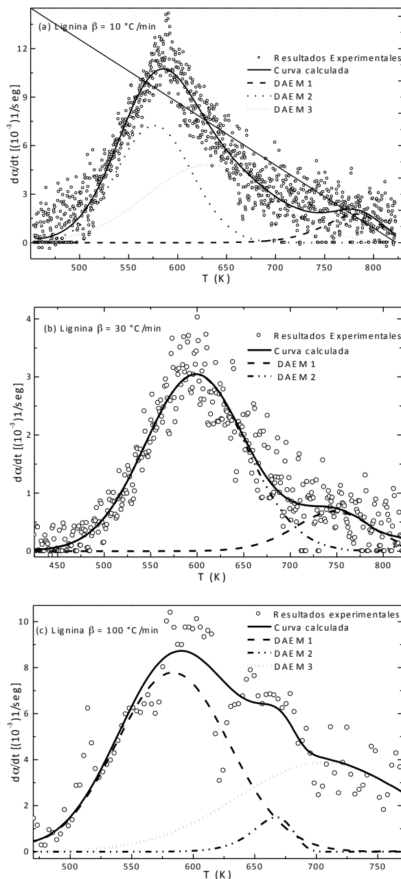
Figura 5. Ajuste del modelo DAEM con diferentes números de conjuntos de reacciones para la pirólisis de la lignina.
