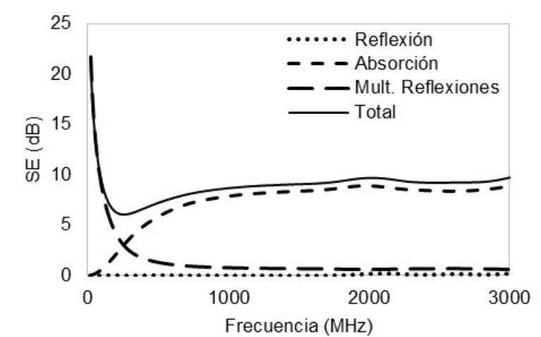
Figura 6. Efectividad de apantallamiento ofrecida por un muro de concreto con 0,15 m de espesor y 1 m de alto.
