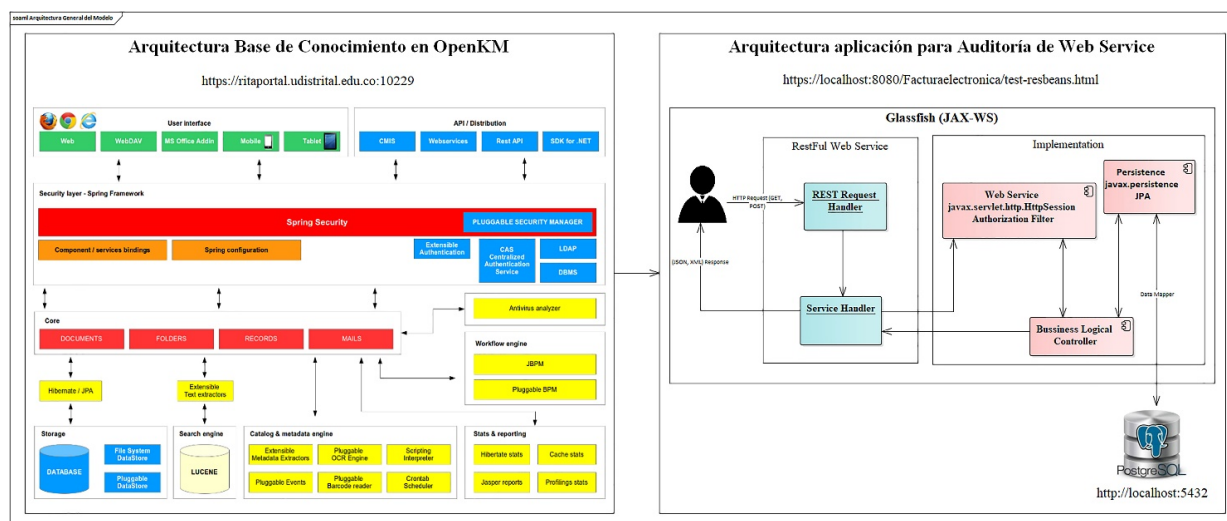
Figura 4. Arquitectura del modelo general Fuente: [14].
