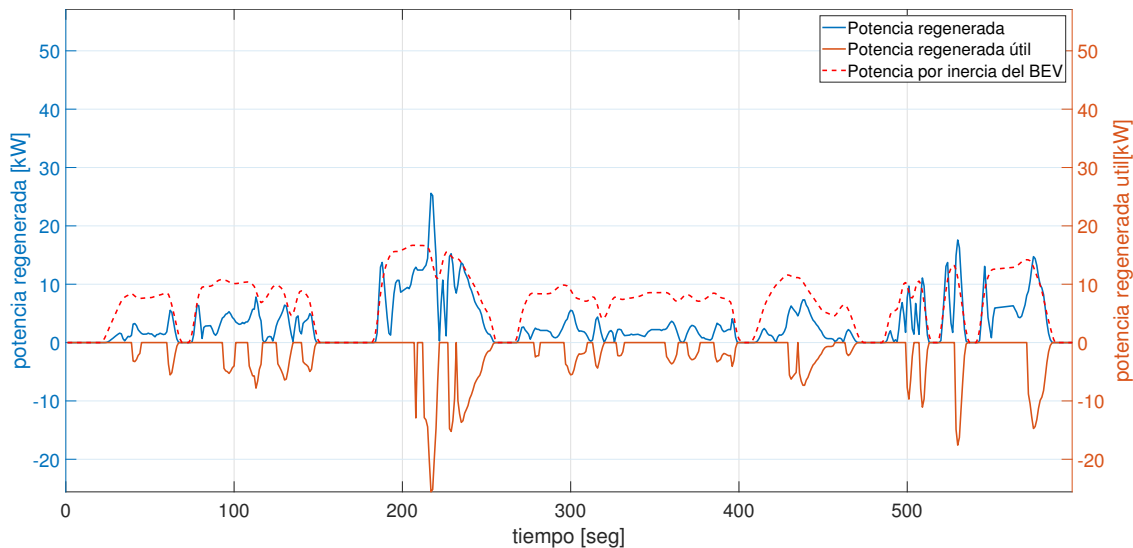
Figura 11. Gráfica de potencia en batería primaria/secundaria con perfil de velocidad traslapado
