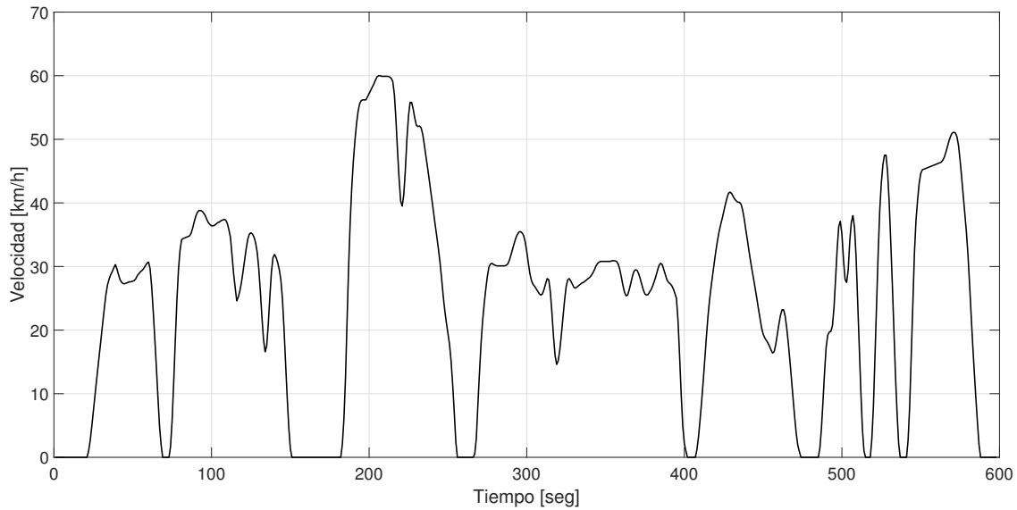
Figura 6. Perfil de velocidad WMTc de baja velocidad [21]
