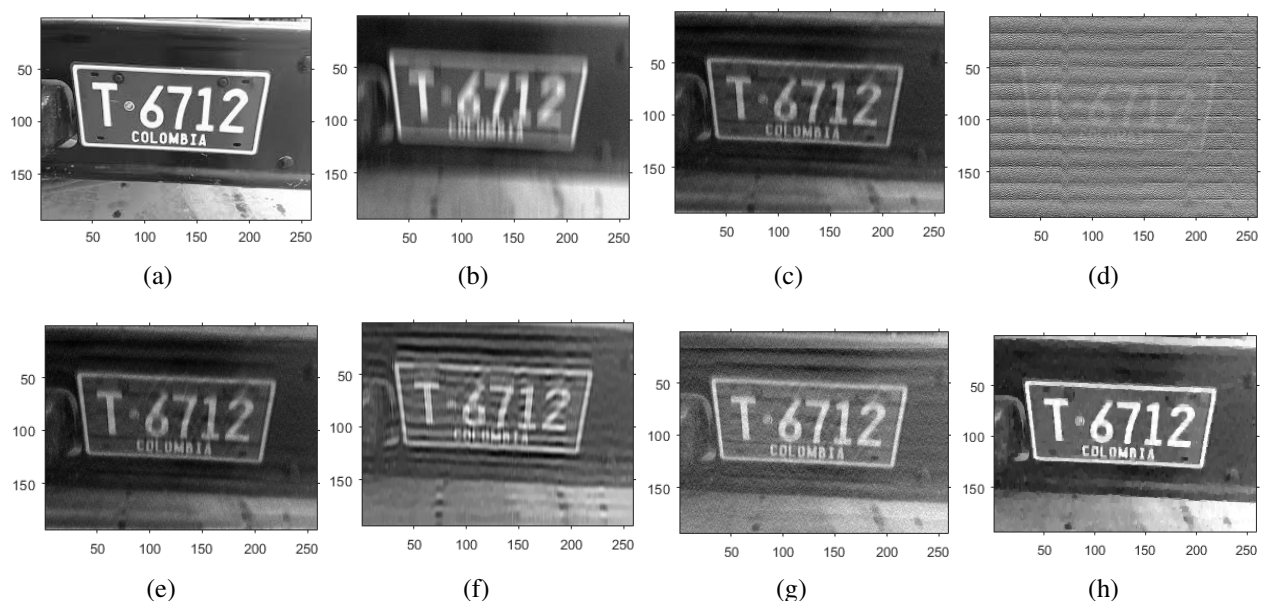
Figura 5. Imagen degradada con 3 % de ruido y sus restauraciones. (a) Imagen original, (b) Imagen borrosa, (c) Imagen restaurada con método de Lucy-Richardson, (d) Imagen restaurada con método de deconvolución de Wiener, (e) Imagen restaurada con el método blind deconvolution , (f) Imagen restaurada con método BDNSM, (g) Imagen restaurada con método de regularización de Tikhonov, (h) Imagen restaurada con método propuesto.
