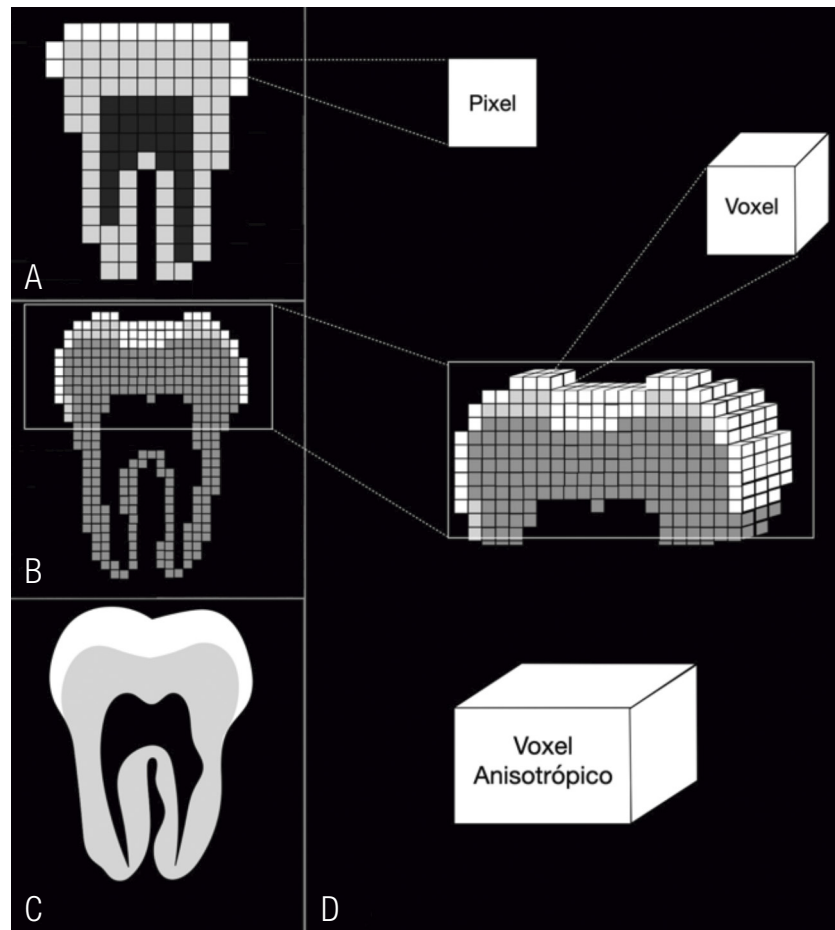
Figura 2. Las imágenes bidimensionales representadas en A, B, C están compuestas por pixels de mayor, medio y menor tamaño, respectivamente, lo que se traduce en resoluciones baja, media y alta. D) Diferencia entre pixel (2D), voxel isotrópico (3D) característico de los equipos CBCT y voxel anisotrópico (3D) más común en los equipos MDCT.
