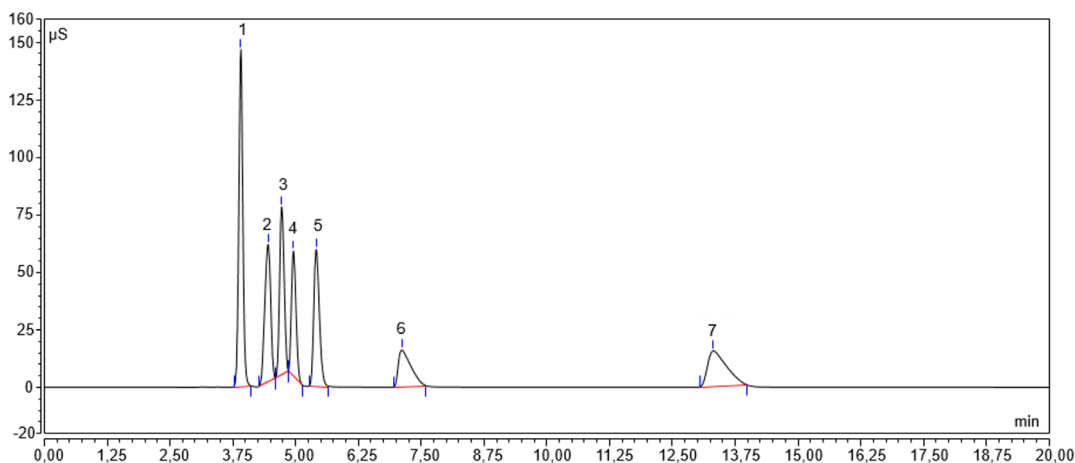
Figura 1. Cromatograma de siete aniones: 1. cloruro, 2. nitrito, 3. sulfato, 4. bromuro, 5. nitrato, 6. fosfato y 7. Tiocianato.
