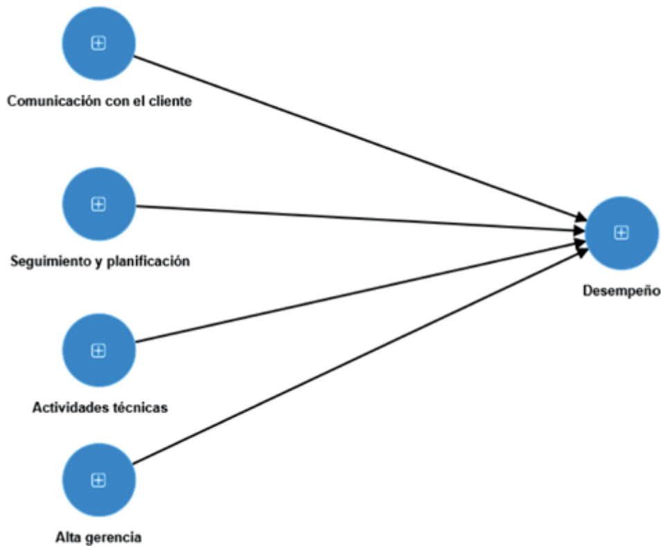
Figura 1 Modelo propuesto
