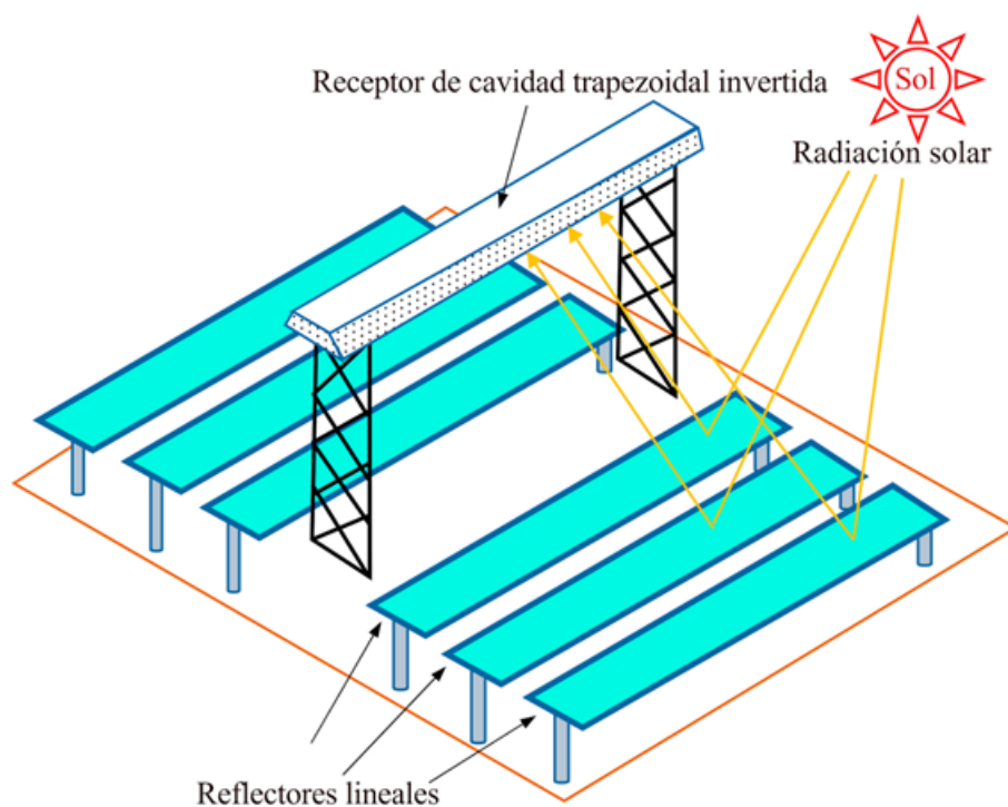
FIGURA 7. Esquema de un colector lineal Fresnel [9]
