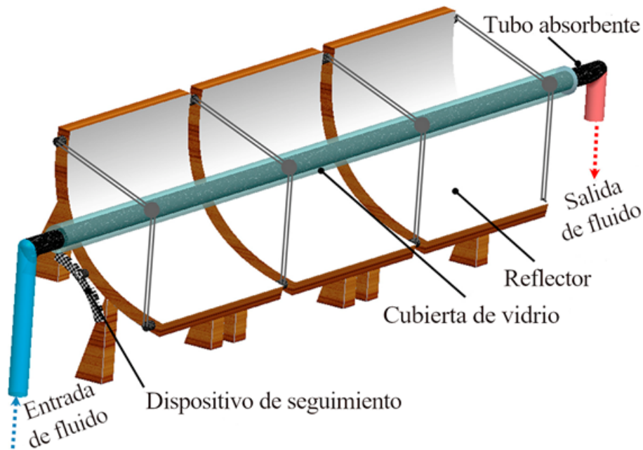
FIGURA 6. Esquema de un colector cilindro parabólico [21]
