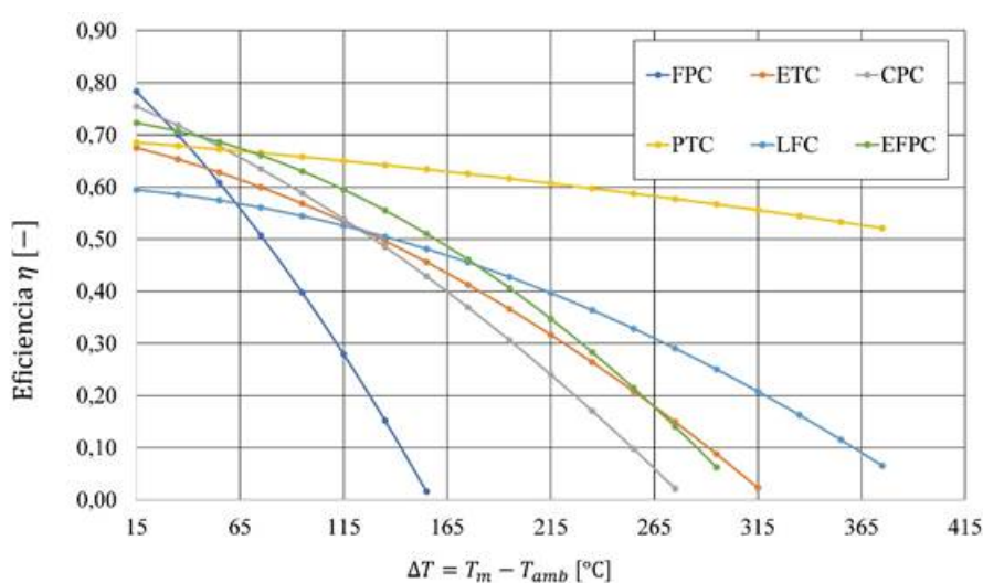
FIGURA 8. Comparativa entre colectores solares
