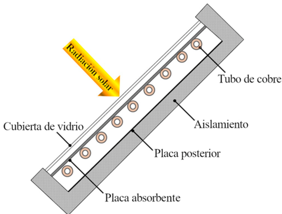
FIGURA 1. Partes de un colector de placa plana [21]
