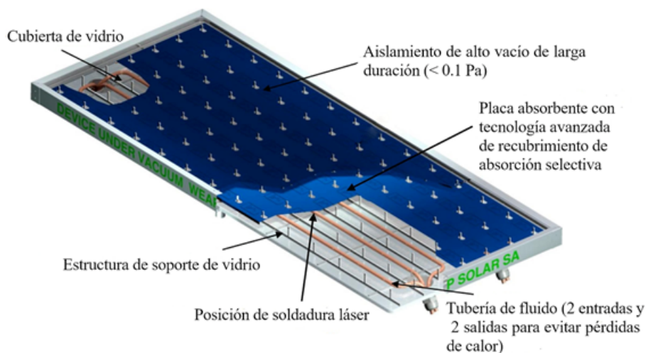
FIGURA 5. Estructura del colector de placa plana evacuado [25]
