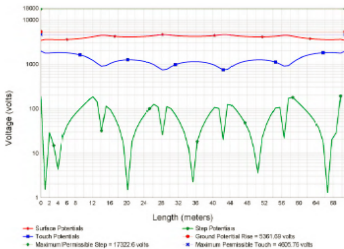
FIGURA 8. Perfil de potencial de la malla aislada- asfalto \rho_s asphalt
