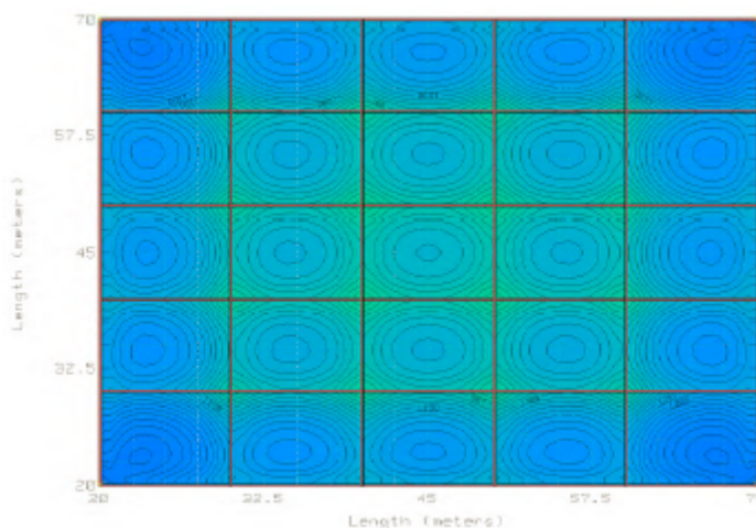
FIGURA 18. Contorno del potencial de malla – sin rieles
