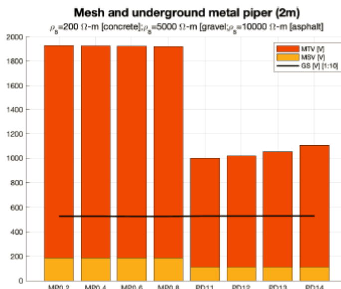
FIGURA 16. Visualización de valores de la Tabla 8
