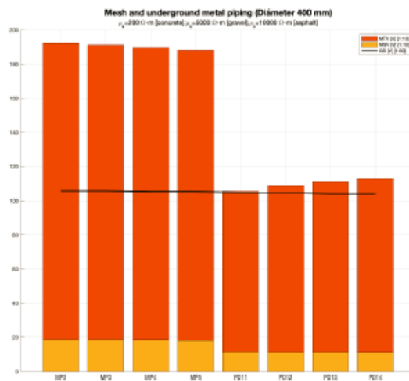
FIGURA 15. Métrica de malla y tubería metálica subterránea
