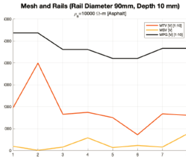
FIGURA 23. Visualización de los valores de la Tabla 6
