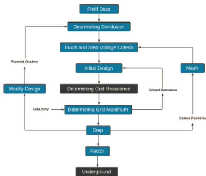
FIGURA 2. Metodología utilizada para el diseño
