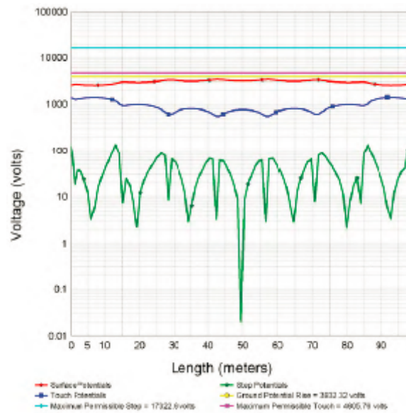
FIGURA 10. Malla de potencial y perfil de la valla sin asfalto-conexión ps
