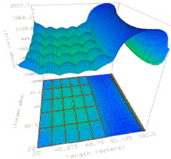
FIGURA 20. Voltaje de contacto para malla y rieles sin conexión
