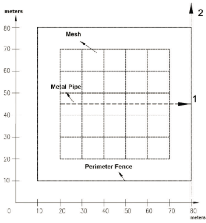
FIGURA 3. Vista superior del GS del caso de estudio 1
