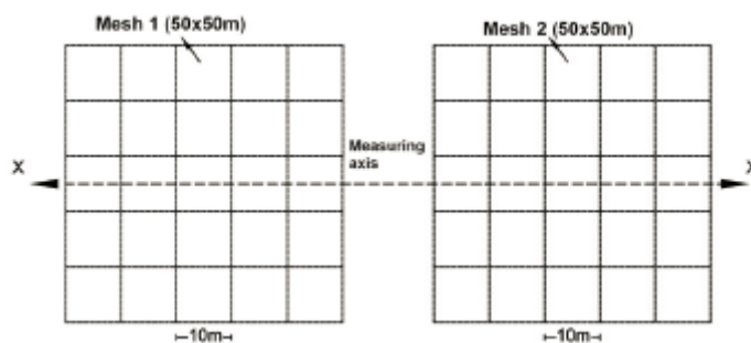
FIGURA 6. Mallas de puesta a tierras cercanas
