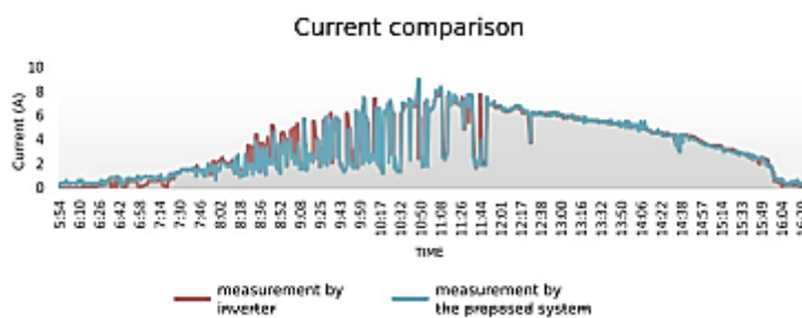
FIGURA 6. Comparación de corriente entre el inversor y el sistema propuesto
