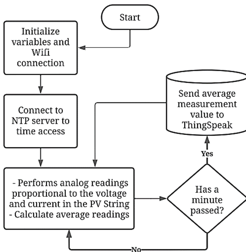
FIGURA 3. Diagrama de flujo del código fuente (firmware)
