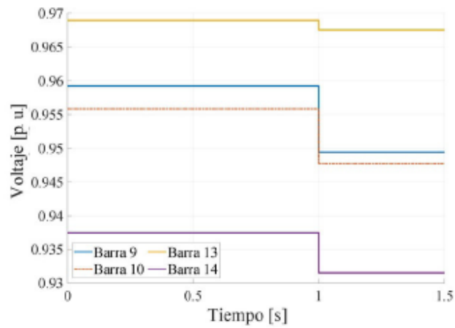
(a) Perfil de tensión
