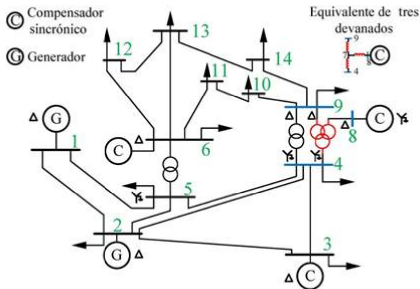
FIGURA 1. Caso base sistema IEEE 14 Barras
