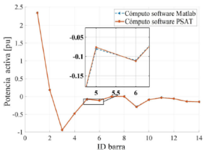
(a) Potencia activa nodal en p. u.
