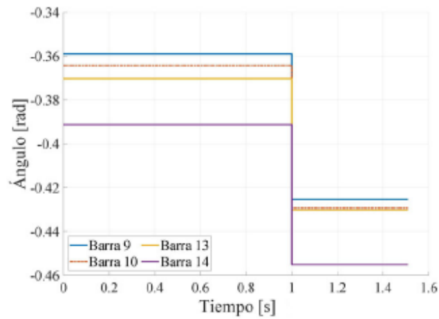
(b) Perfil de ángulo
