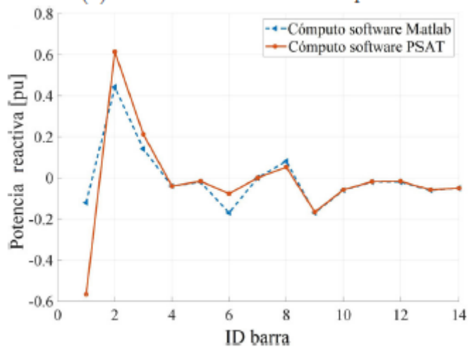
(b) Potencia reactiva nodal en pu
