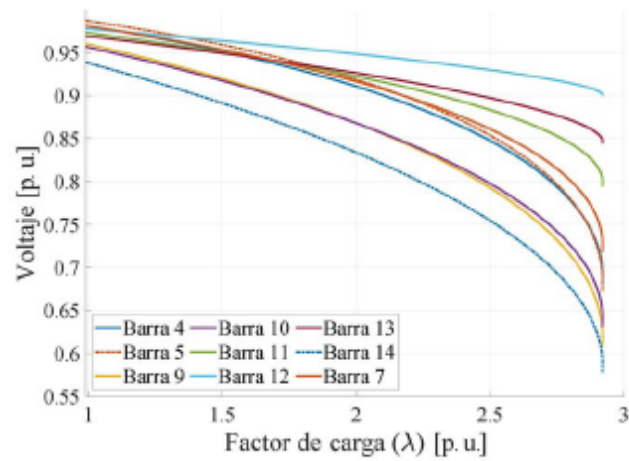
(a) Curva PV en condiciones normales
