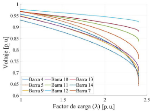
(b) Curva PV en contingencia N - 1
