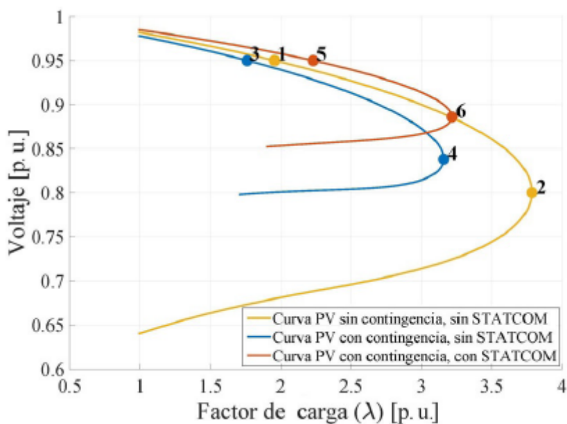
FIGURA 5. Nivel de tensión en función de parámetros normales de operación, contingencia N-1 utilizando compensación reactiva
