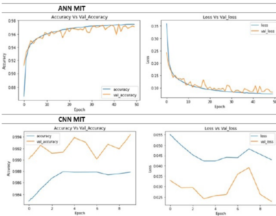
FIGURA 7. Exactitud vs. Pérdida para cada uno de los algoritmos sobre el conjunto de datos MIT
