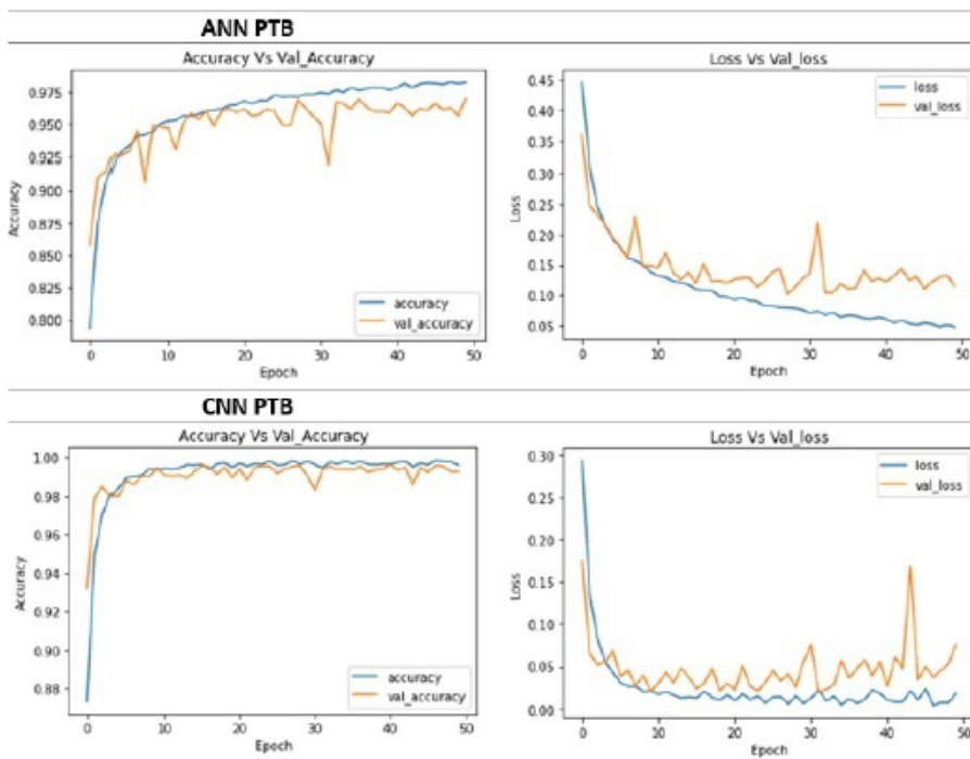
FIGURA 6. Exactitud vs. Pérdida para cada uno de los algoritmos sobre el conjunto de datos PTB
