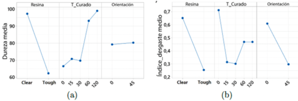
Figura 6. Gráfico de efectos principales. a) Dureza, b) Resistencia a la abrasión - Prueba Tabber
