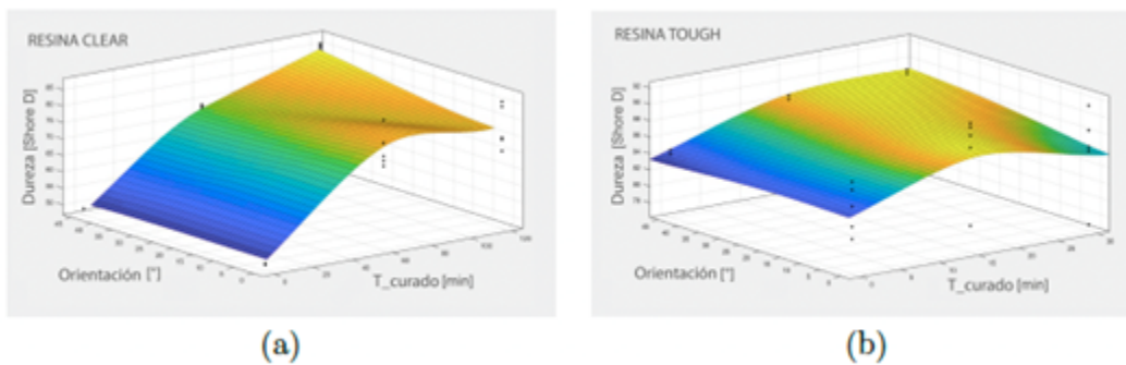
Figura 7. Resultados experimentales. (a) Resina Clear: Dureza vs. Orientación vs. Poscurado (b) Resina Tough: Dureza vs. Tiempo de poscurado vs. Orientación
