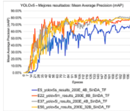
Figura 9. YOLOv5 – Mejores resultados: mAP –Entrenamiento del modelo
