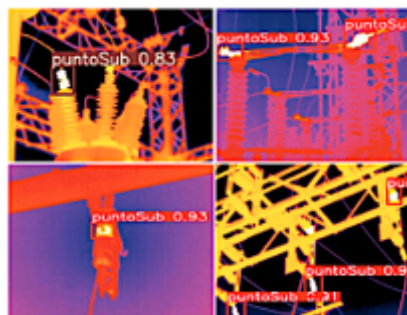
Figura 15. YOLOv5 medium – Detección de puntos calientes
