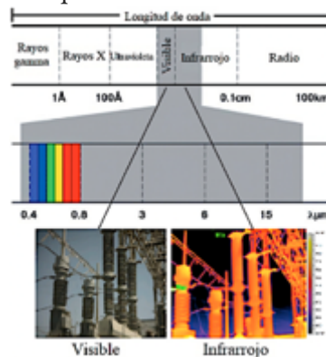
Figura 6. Espectro electromagnético de una subestación eléctrica
