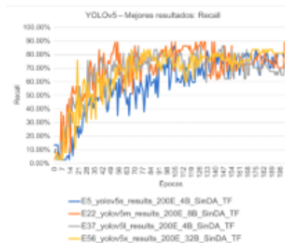
Figura 11. YOLOv5 – Mejores resultados: Recall – Entrenamiento del modelo
