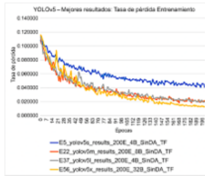
Figura 12. YOLOv5 – Mejores resultados: Tasa de pérdida – Entrenamiento del modelo
