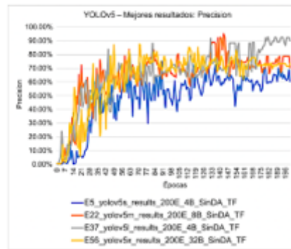
Figura 10. YOLOv5 – Mejores resultados: Precision – Entrenamiento del modelo
