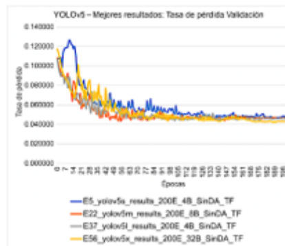
Figura 13. YOLOv5 – Mejores resultados: Tasa de pérdida – Validación del modelo
