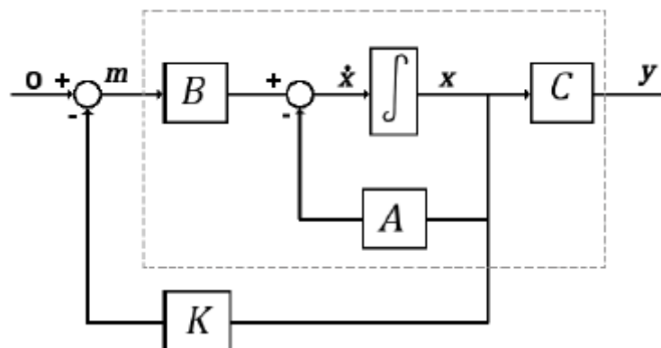
FIG. 4. ESQUEMA DE UN LQR.
