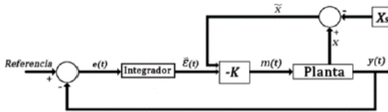
FIG.5. Esquema del controlador LQR+Integral (LQI).
