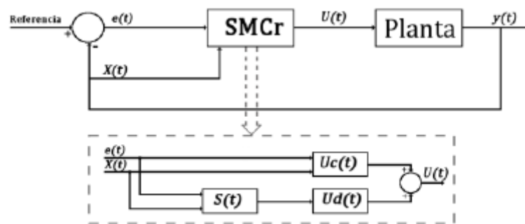
FIG. 3. Esquema controlador SMC.
