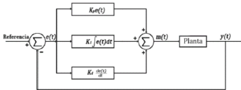
FIG. 1. Esquema controlador PID.
