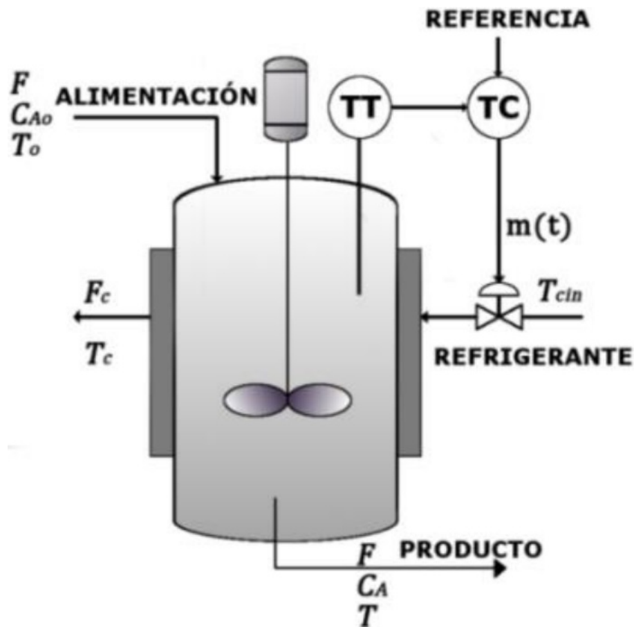
FIG. 16. Reactor con varios puntos de operación.
