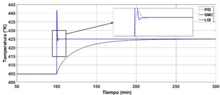
FIG. 17. Respuesta ante cambio de referencia a 425°K.
