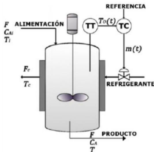
FIG.6. Esquema del Reactor de Dinámica Lenta.
