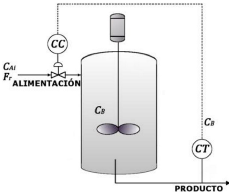
FIGURA 11. Reactor Van de Vusse, respuesta con respuesta inversa.
