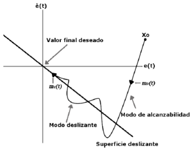
FIG.2. Representación gráfica de un SMC.
