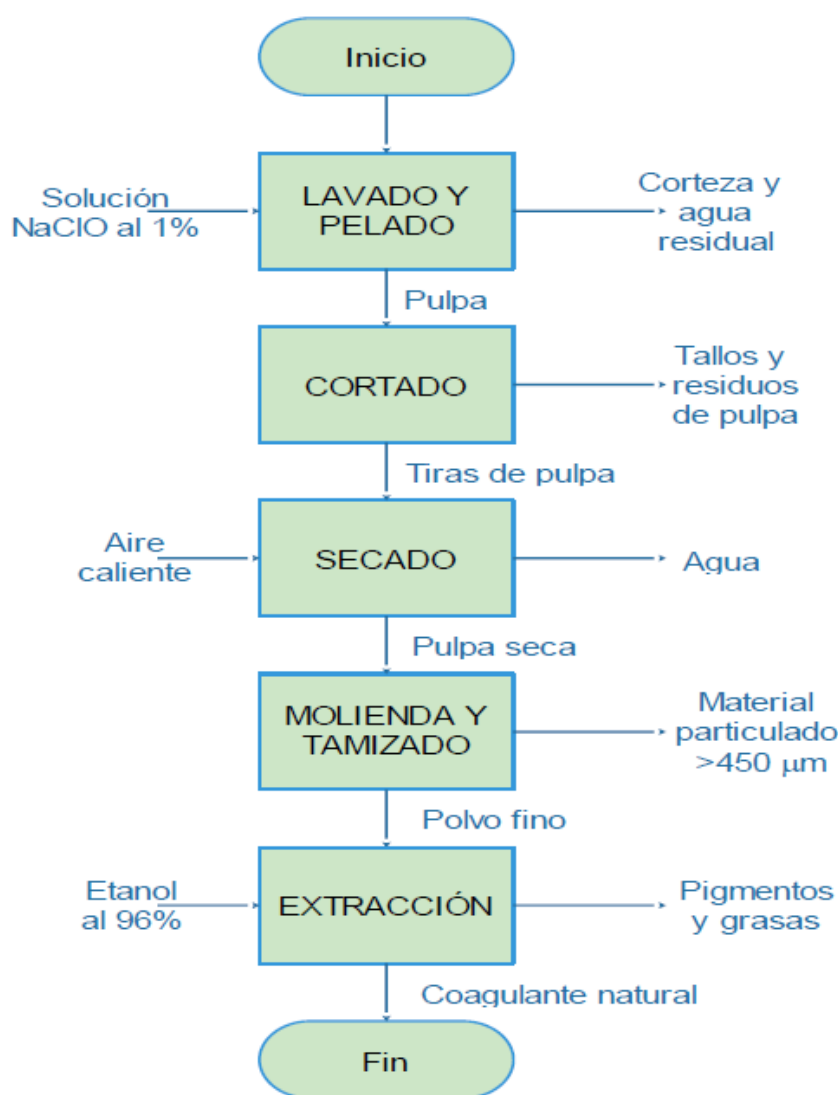
FIG. 1 Procedimiento para la obtención del coagulante
