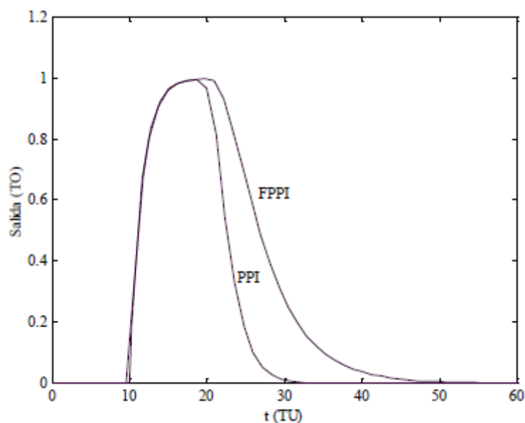
FIGURA 12 Respuestas de los sistemas ante una perturbación
