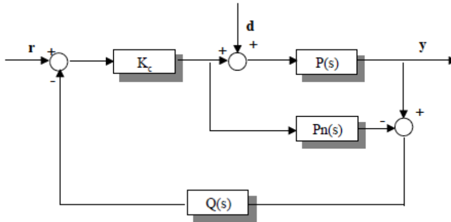
FIGURA 5 Controlador FPPI
