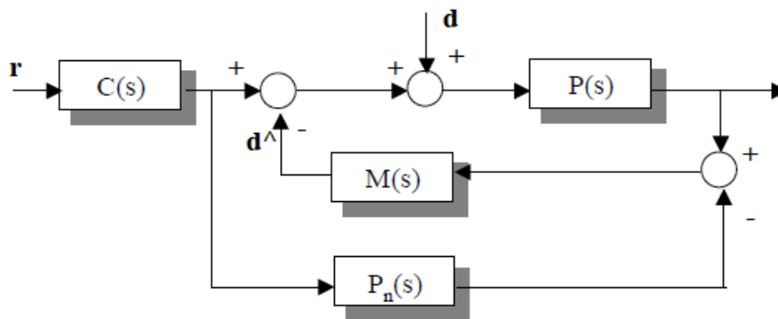
FIGURA 4 DTC modificado por Zhang et. al.
