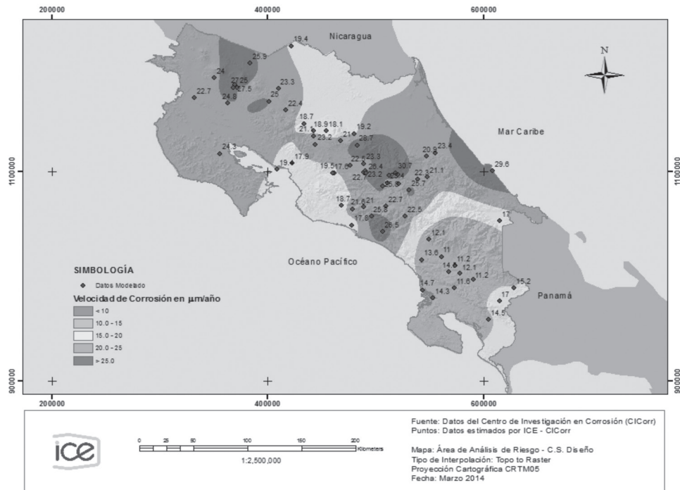
Fig. 7. Corrosión Atmosférica para acero de baja aleación según Modelado de la ISO 9223:2012 ( \mu\text{m}\cdot\text{año}^{-1} ).
