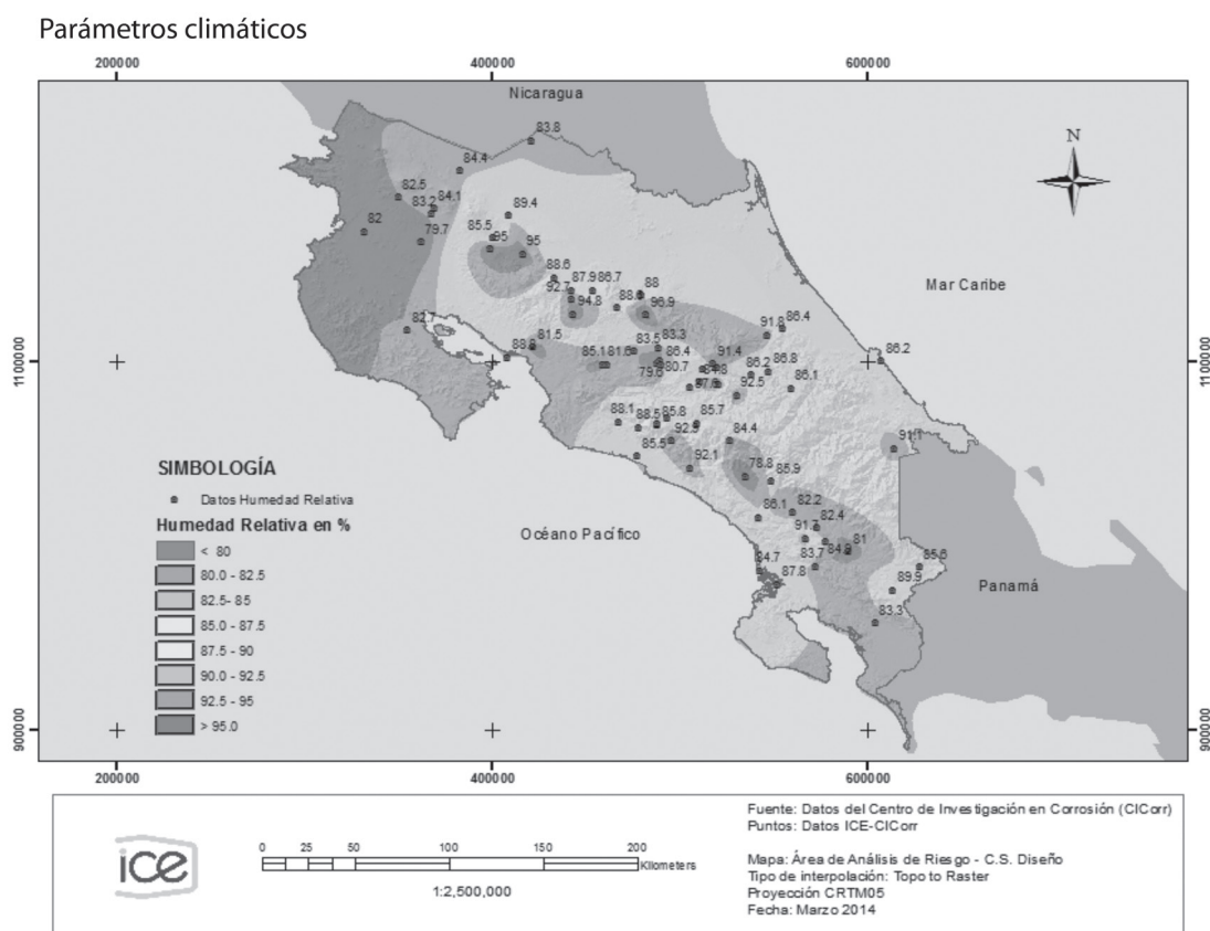
Fig. 1. Humedad Relativa Media Anual (%).
