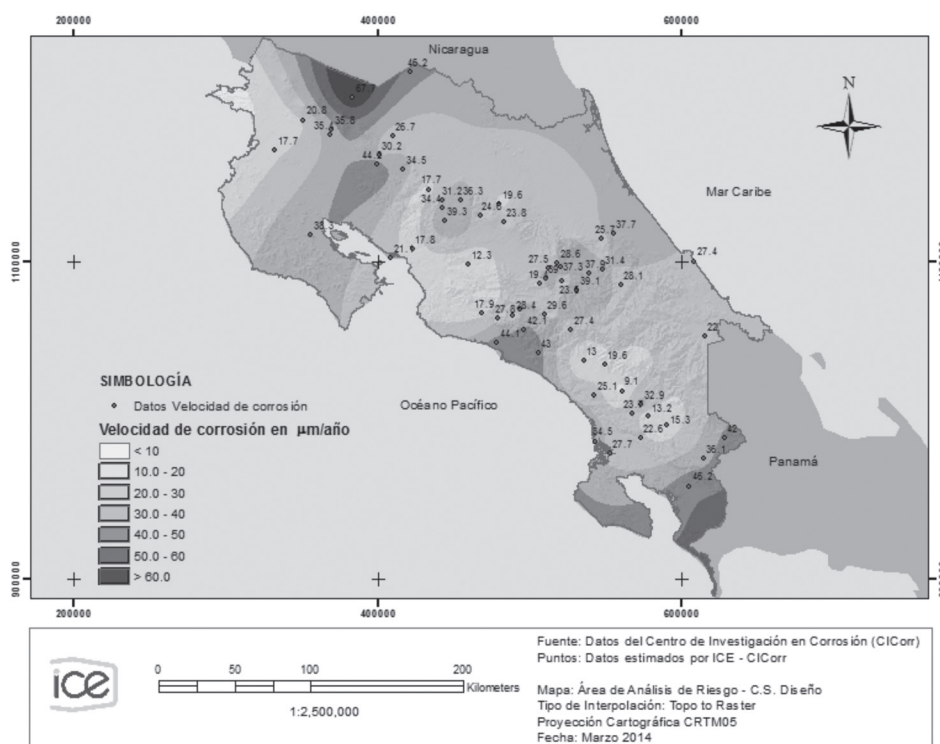
Fig. 8. Corrosión Atmosférica para acero de baja aleación según Modelado lineal con un año de mediciones del CICorr, en base a \text{Cl} , \text{SO}_2 y \text{TDH} ( \mu\text{m}\cdot\text{año}^{-1} ).
