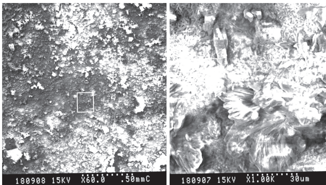
Fig. 3. Microscopia de acero ASTM A36 luego de un año de exposición en el Centro Geotérmico Las Pailas, a) barrido general, b) detalle con óxidos de Goethita .
