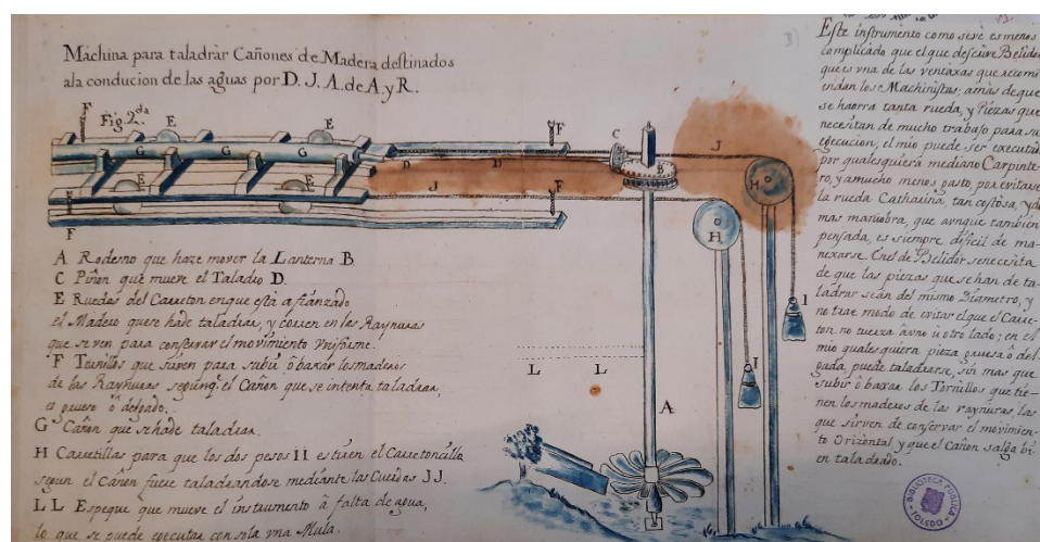
Imagen 4. Invento para taladrar madera con que hacer las cañerías de abasto de agua en la ciudad de México. Papeles relativos al gobierno político, económico y civil de Indias . BCLM, Fondo Histórico, ms. 22, doc. 2
