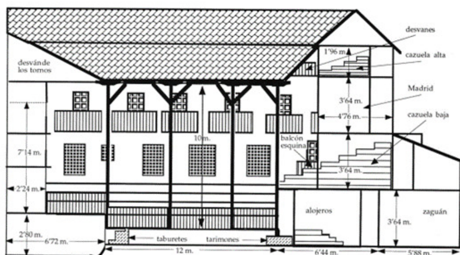
Imagen 5: Corte transversal del corral del Príncipe siguiendo la propuesta de Allen, e indicando medidas de las estancias del edificio. Fuente: Ferrer Valls, Teresa, Diccionario biográfico de actores del teatro clásico español (DICAT) , Kassel, Edition Reichenberger, 2008.
