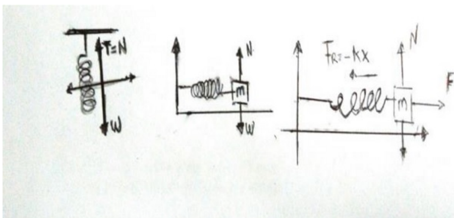
Figura 2 Diagrama de cuerpo libre
