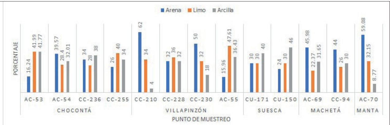
Figura 3 Granulometría Almeidas
