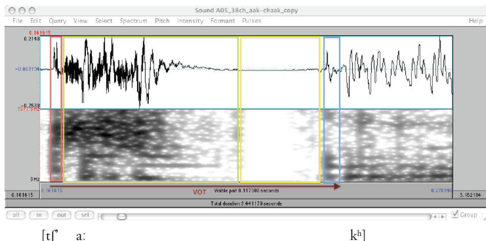
Figura 11. Oscilograma y espectrograma de /tʃʰa:kʰ/ ‘rebanar’
