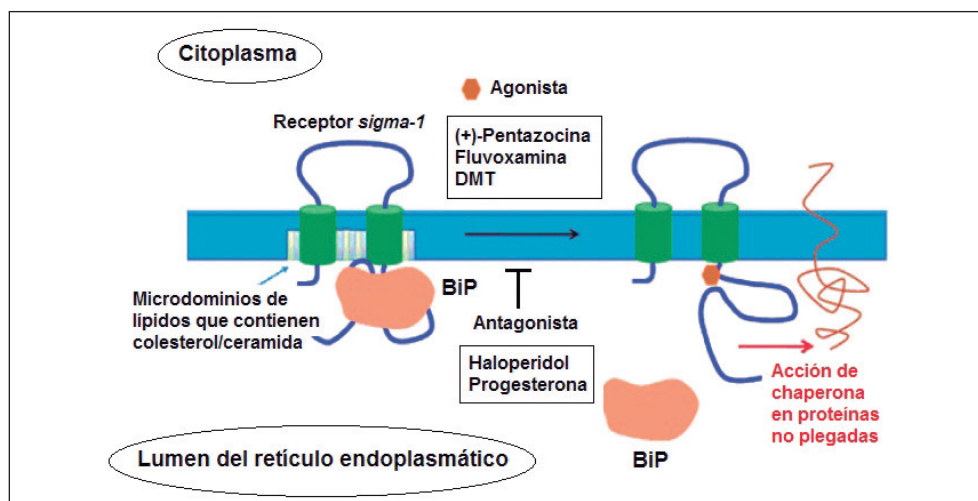
Figura 8. El receptor chaperona sigma-1 tiene regulación operada por ligando y es sensible a \text{Ca}^{2+} . Los agonistas de sigma-1 (como DMT) o la depleción de \text{Ca}^{2+} del retículo endoplasmático disocian sigma-1 de BiP, lo cual conduce a una prolongada señalización de \text{Ca}^{2+} en las mitocondrias a través de los receptores de trifosfato de inositol ( \text{IP}_3 ). La unión de DMT a los receptores sigma-1 permite explicar el diferente comportamiento que este compuesto presenta in vivo en el cerebro, en comparación con triptamina y serotonina. Además, sigma-1 está implicado en la neuroprotección, la carcinogénesis y la neuroplasticidad.
