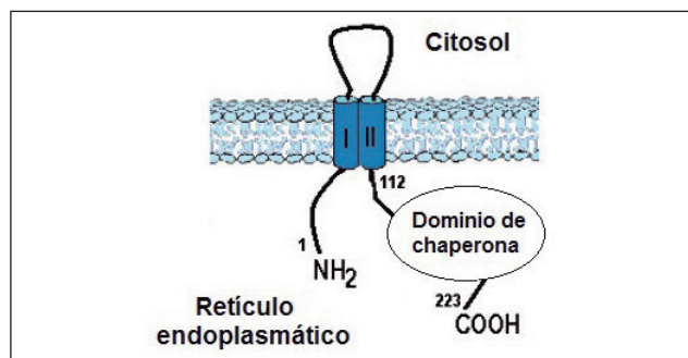
Figura 7. Topología del receptor sigma-1 . Se observan dos hélices de transmembrana ( \text{TM}_1 y \text{TM}_2 ), indicadas como I y II, y el dominio asociado a la membrana. Se indican los extremos N y C (N- y C-terminales) y las posiciones aproximadas de los residuos 112 y 223 (residuo C-terminal).
