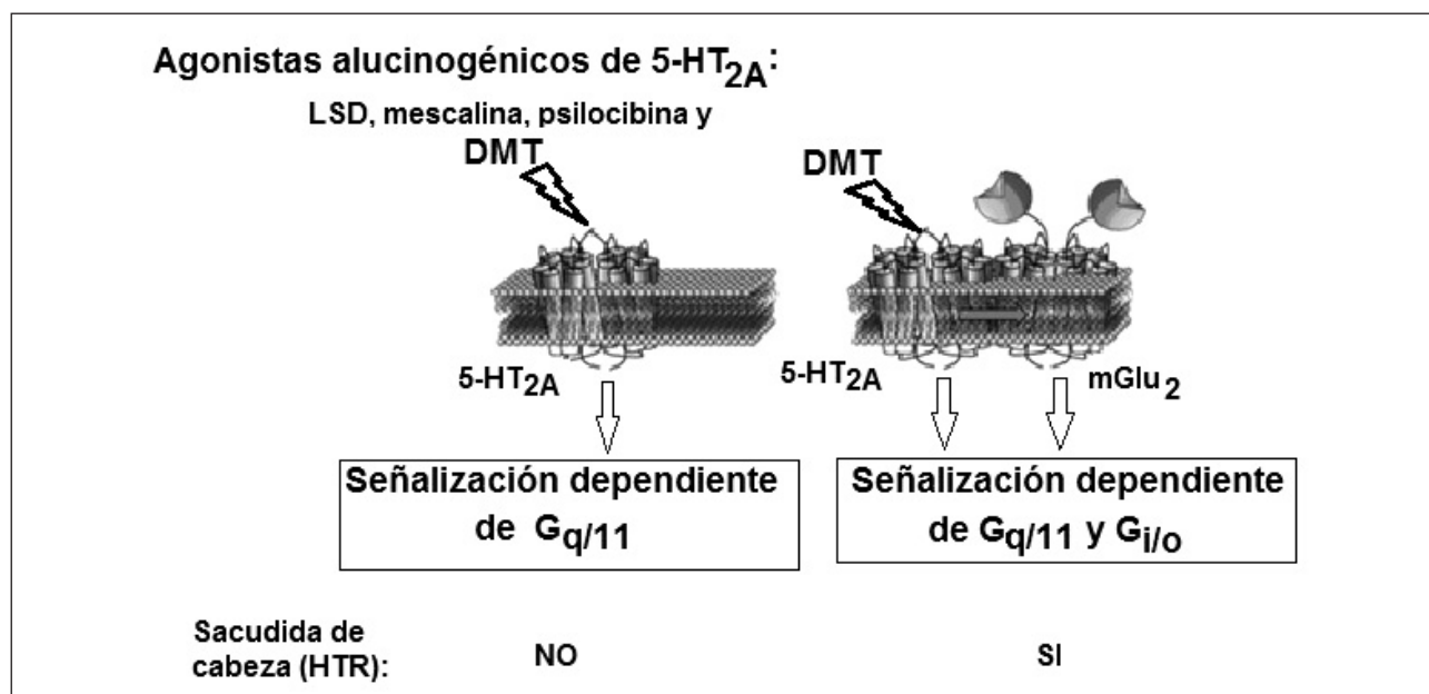
Figura 9. Importancia del heterocomplejo funcional mGlu 2 -5-HT 2A en la corteza cerebral (y en cultivos de tejidos). A través de este complejo los ligandos de serotonina y de glutamato modulan el patrón de acoplamiento de las proteínas G en las células vivas. Sacudida de cabeza de ratones: respuesta conductual provocada por alucinógenos: A: Ausente en ratones 5-HT 2A -KO y en ratones mGlu 2 -KO. B: Hay respuesta en presencia del complejo mGlu 2 -5-HT 2A . Se necesita el heterocomplejo para la alucinación (demostrado in vivo ).
