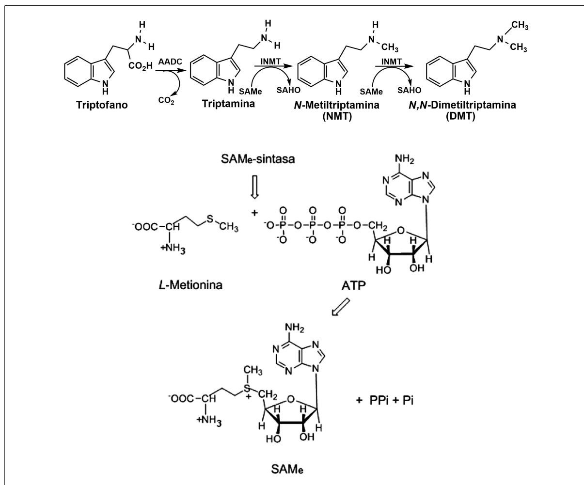
Figura 4. Biosíntesis de DMT a partir del aminoácido triptofano: 1) La descarboxilasa de aminoácidos aromáticos (AADC: del inglés aromatic amino acid decarboxylase ) cataliza la formación de triptamina a partir de triptofano; 2) la indoletilamina-N-metiltransferasa (INMT) transfiere un grupo metilo de SAMe (S-adenosilmetionina) a triptamina, dando N-metiltriptamina (NMT); 3) se repite la reacción anterior con NMT como sustrato, INMT transfiere otro grupo metilo y produce DMT y dos equivalentes de SAHO (S-adenosilhomocisteína) en total.
