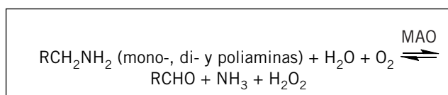
Figura 5. Reacción catalizada por las enzimas monoaminooxidasas (MAO).
