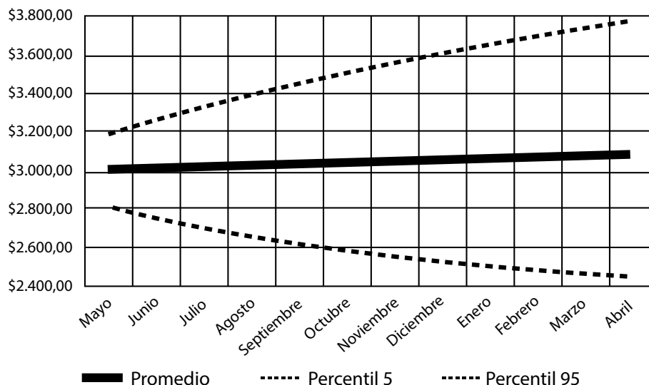
Figura 1. Proyección TRM.
