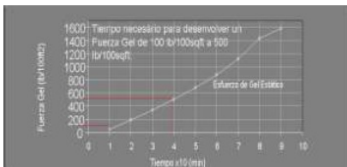
Figura 3. Esfuerzo de Gel Estático. Fuente: Prueba de Laboratorio.
