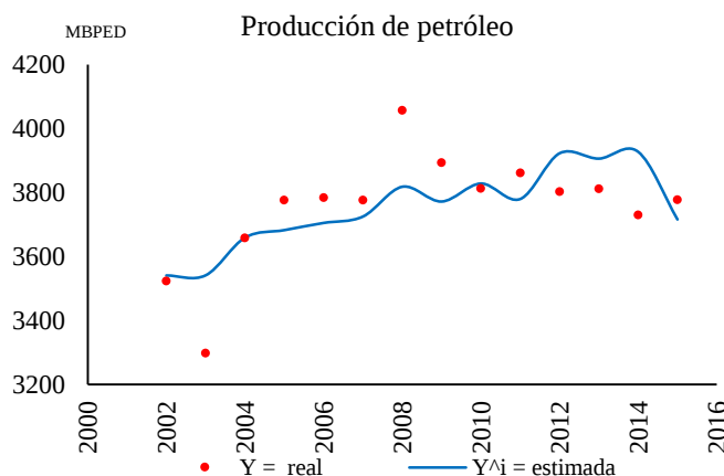
Figura 6. Función de la regresión. Fuente: elaboración propia
