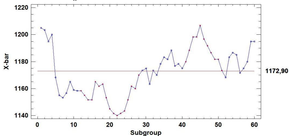
Figura 12. Grafico de promedios Aval primer trimestre, sin límites de control.
