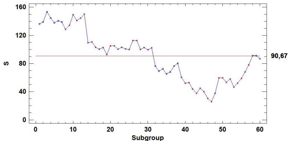
Figura 13. Grafico de desviaciones estándar Aval primer trimestre, sin límites de control.
