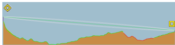
Figura 7. Perfil de elevación y línea de vista Enlace 3: repetidora Cerro Almagra - La Ceiba. Fuente: imagen generada por Radio Mobile.
