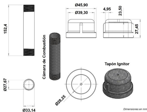
Figura 3. Diseño de la cámara de combustión del motor cohete: planos de fabricación. Fuente: elaboración propia.
