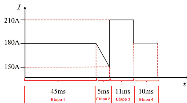
Figura 12. Optimización de forma de onda en corriente pulsada. Fuente: adaptado de [48].
