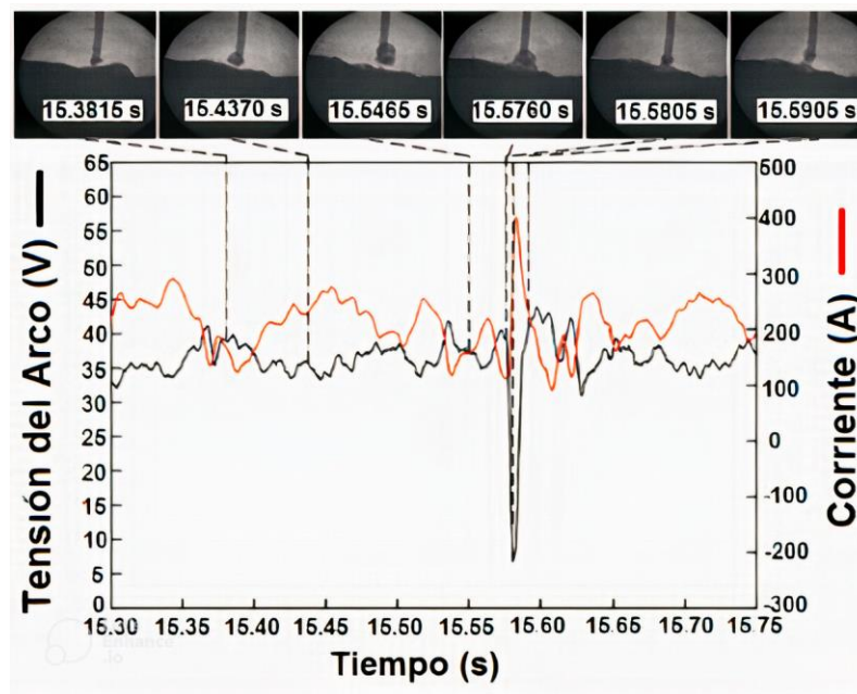
Figura 3. Imágenes capturadas a alta velocidad (superior) y oscilogramas de tensión y corriente (inferior) evidenciados en transferencia de tensión superficial. Fuente: adaptado de [33].
