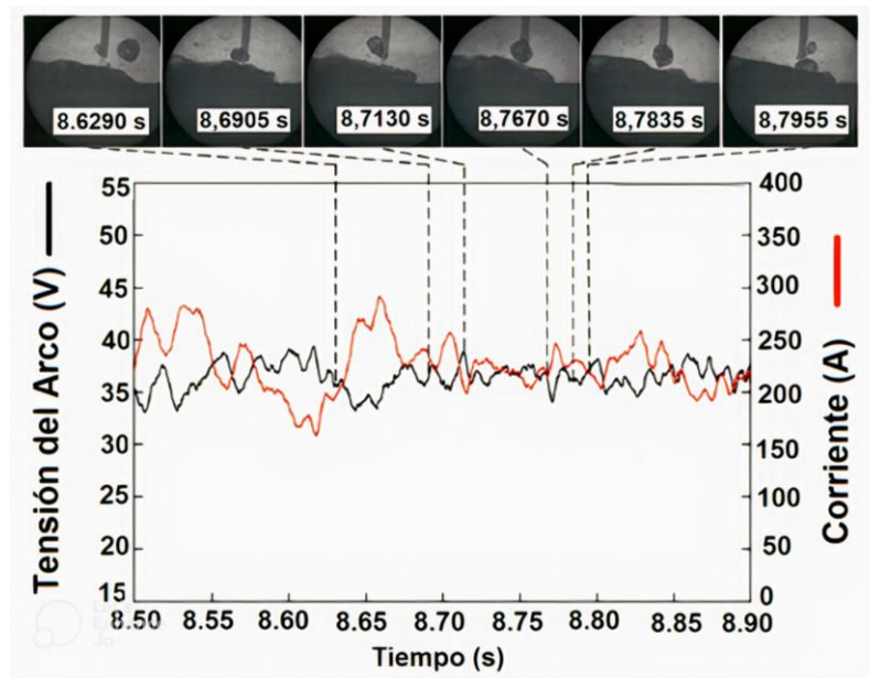
Figura 2. Imágenes capturadas con filmación de alta velocidad (superior) y oscilogramas de tensión y corriente (inferior) evidenciados en transferencia repelida de ángulo agudo. Fuente: adaptado de [33].
