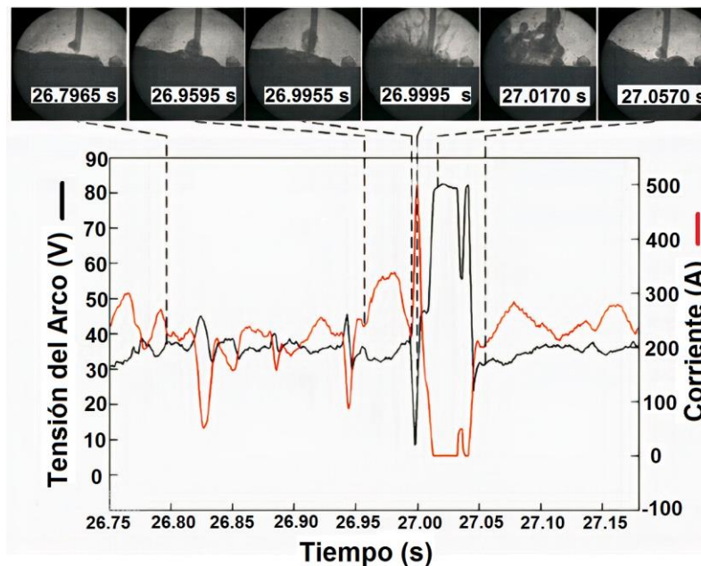
Figura 4. Imágenes capturadas con filmación de alta velocidad (superior) y oscilogramas de tensión y corriente (inferior) evidenciados en transferencia explosiva. Fuente: adaptado de [33].
