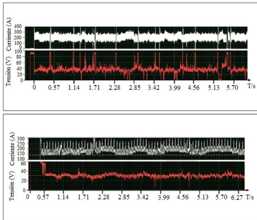
Figura 9. Señales de corriente de y tensión recolectadas del alambre tubular usado en soldadura submarina usando corriente antes (superior) y después (inferior) de la aplicación del control de longitud del arco. Fuente: adaptado de [47] .
