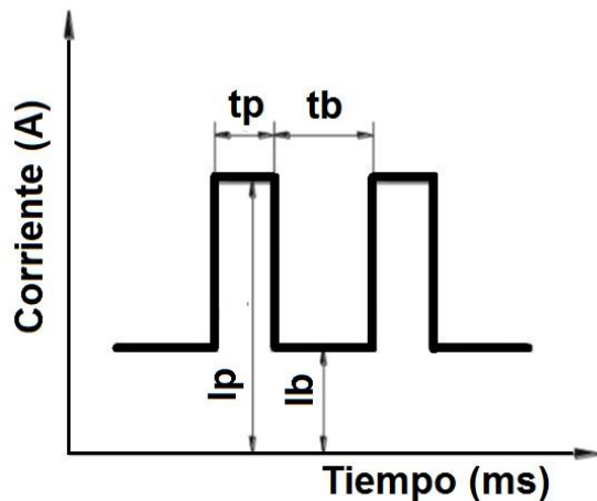
Figura 7. Variables en corriente pulsada: tp – Tiempo de pico; tb – Tiempo de base; Ip – Corriente de pico; Ib – Corriente de base. Fuente: adaptado de [38].
