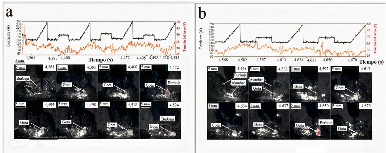
Figura 10. Transferencia metálica típica en soldadura húmeda con alambre tubular utilizando corriente pulsada. Fuente: adaptado de [47].
