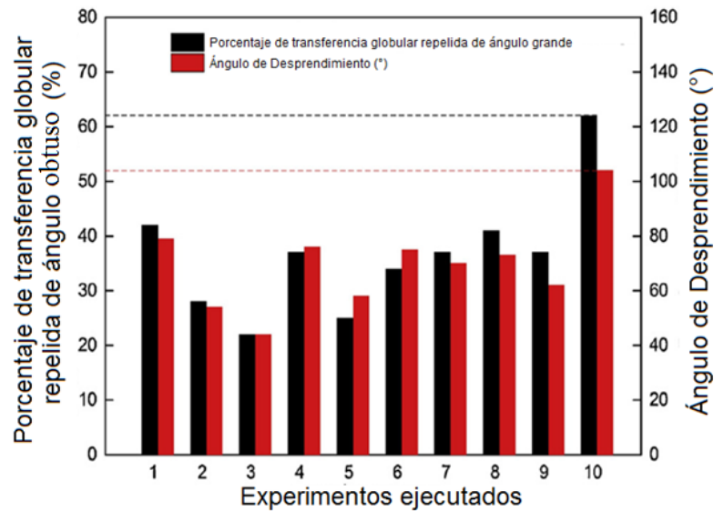
Figura 8. Ángulo de desprendimiento y porcentaje de transferencia globular repelida de ángulo obtuso para los experimentos de soldadura con alambre tubular. Fuente: adaptado de [44] .
