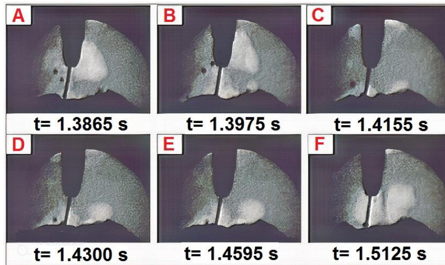
Figura 5. Imágenes capturadas con filmación de alta velocidad evidenciando transferencia de arco sumergido. Fuente: adaptado de [27].
