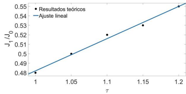
Figura 6. J_1 en función de \tau . Resultados teóricos (puntos negros) y ajuste lineal (línea azul).
