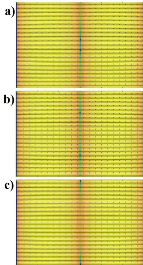
Figura 4. Logaritmo del parámetro de orden ( \ln \psi ) para la muestra homogénea \tau = 1;05 . Color amarillo (azul) corresponde a valores de cerca de 1(0) . Las flechas negras identifican las supercorrientes.
