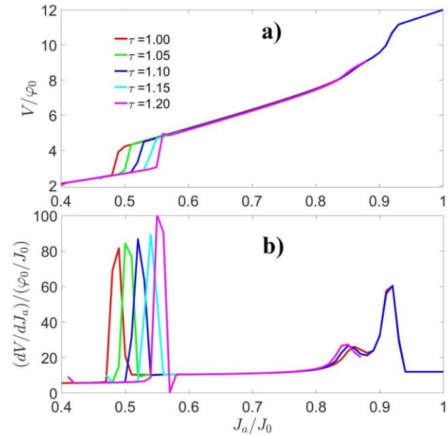
Figura 2. Voltaje V promediado en el tiempo en función de la densidad de corriente aplicada J_a para varias alturas del pilar \tau = 1; 0.0; 1.05; 1.10; 1.15; 1.20 . (b) Resistividad \partial V / \partial J_a en función de la corriente aplicada J_a .
