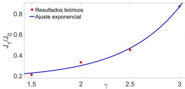
Figura 8. Corriente crítica J_1 en función de \gamma ; para \tau = 1;1 . Resultados teóricos (Puntos rojos) y su respectivo ajuste exponencial (Línea azul).
