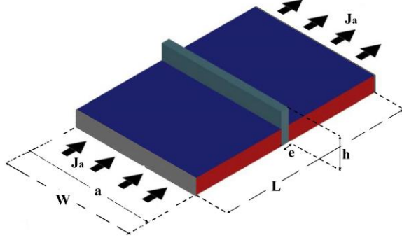
Figura 1. Esquema de la muestra estudiada. Película superconductora de ancho W = 8\xi , largo L = 12\xi , con un pilar central rectangular de base e = 1\xi y altura h . La muestra está en presencia de una corriente continua J_a aplicada a través de los electrodos metálicos de ancho a = W . h es simulado mediante la función \tau ; h = 0 para \tau = 1 , h > 0 para \tau > 1 .
