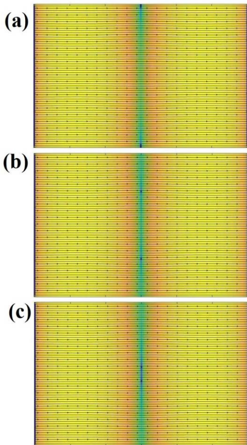
Figura 5. Logaritmo del parámetro de orden ( \ln \psi ) para la muestra homogénea \tau = 1;20 . Color amarillo (azul) corresponde a valores de cerca de 1(0). Las flechas negras identifican las supercorrientes.
