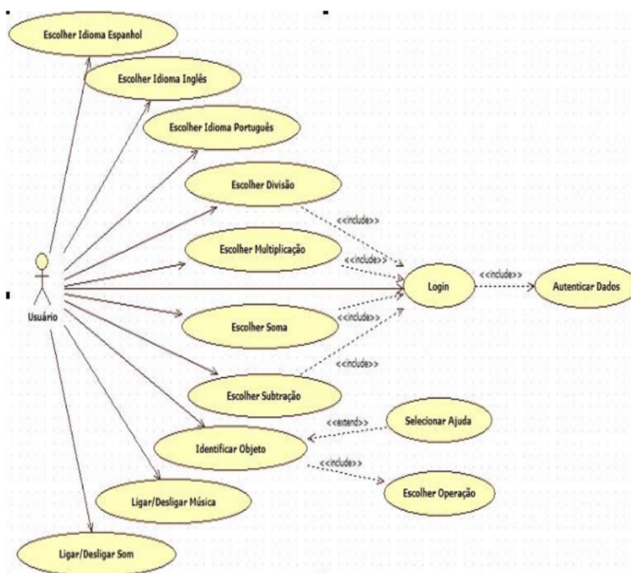
Figura 01 Diagrama de casos de uso Fonte: Elaborada pelos autores
