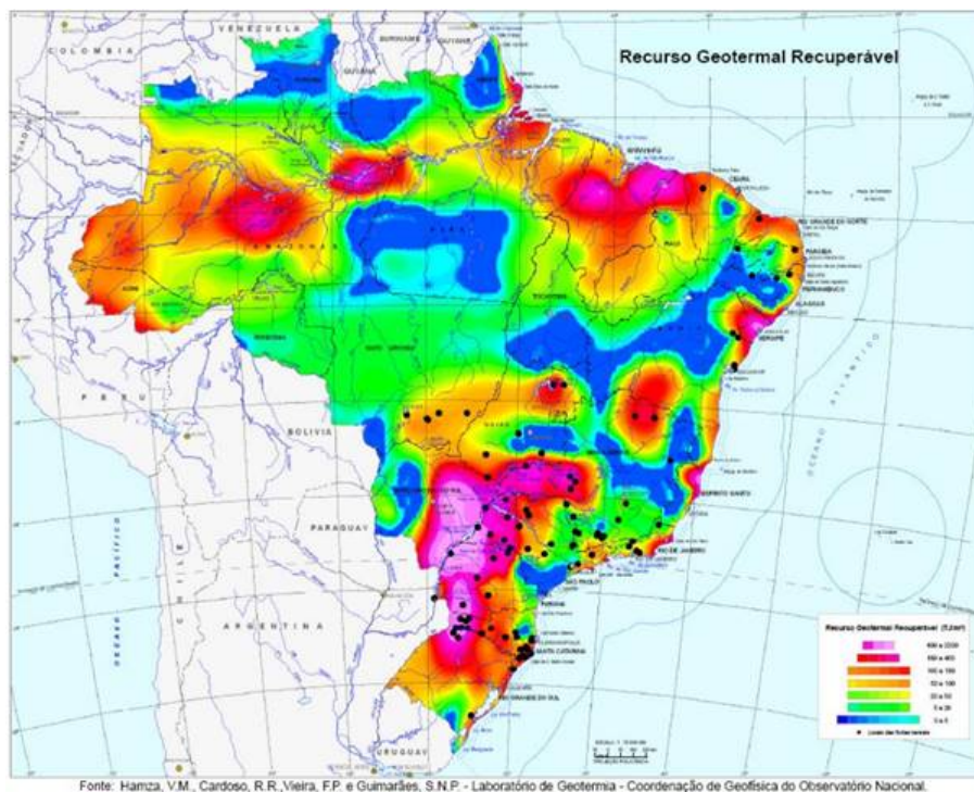
Figura 2 - Mapa de Recurso Geotermal Recuperável.
