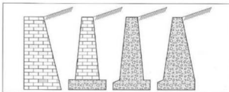
Figura 2 - Muro de Arrimo de Gravidade
