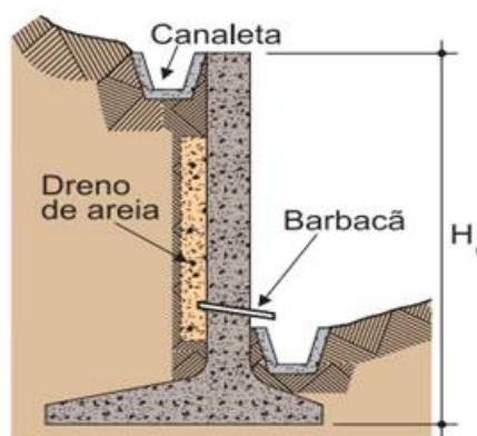
Figura 1- Muro de flexão
