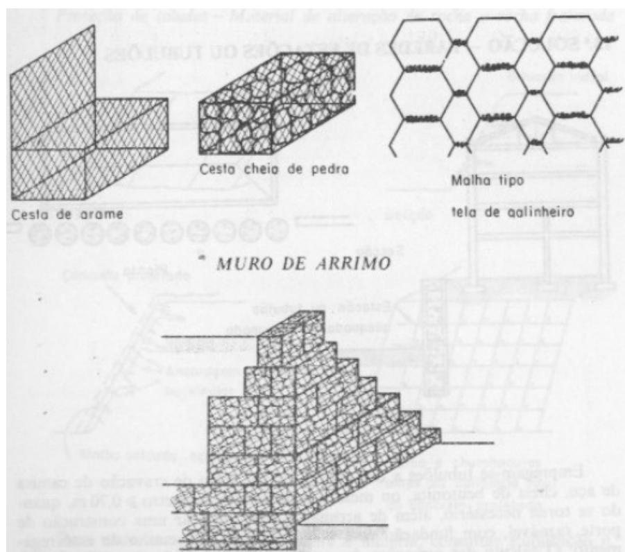
Figura 3- Muro Arrimo de Gabião Fonte: Adaptado Moliterno, 1994.
