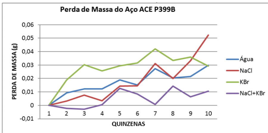
Gráfico 2- Perda de massa do aço ACE P399B. Autor
