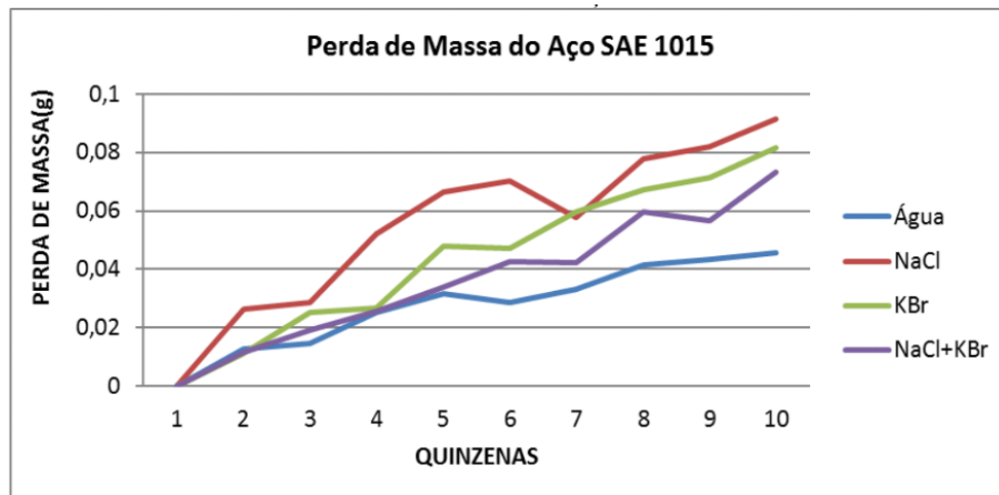
Gráfico 1- Perda de massa do aço SAE 1015. Autor
