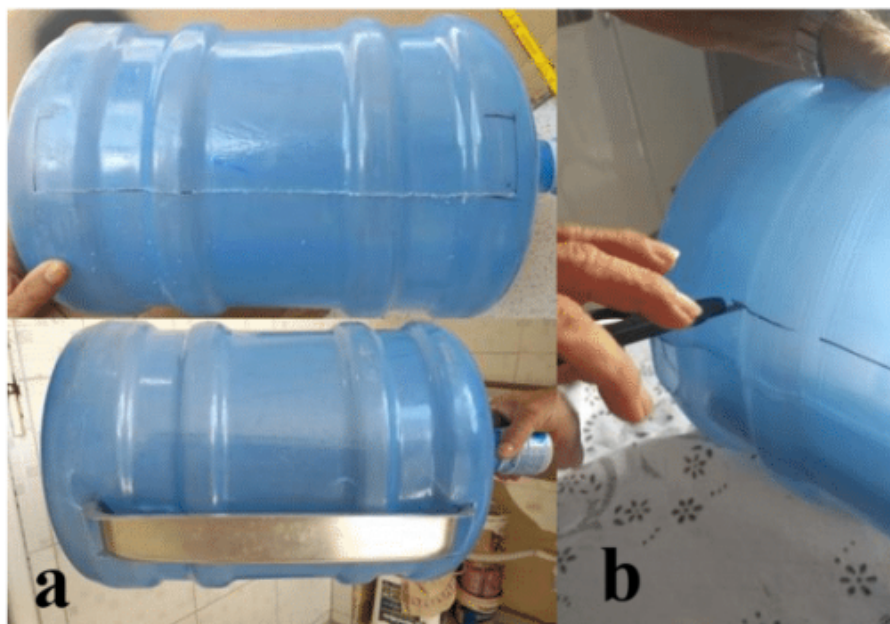
Figura 3. Corte e encaixe da bandeja e furo para o seu suporte Autores (2019)
