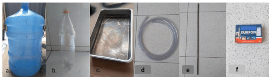
Figura 1. Materiais necessários para produção do destilador solar. Autores (2019)
