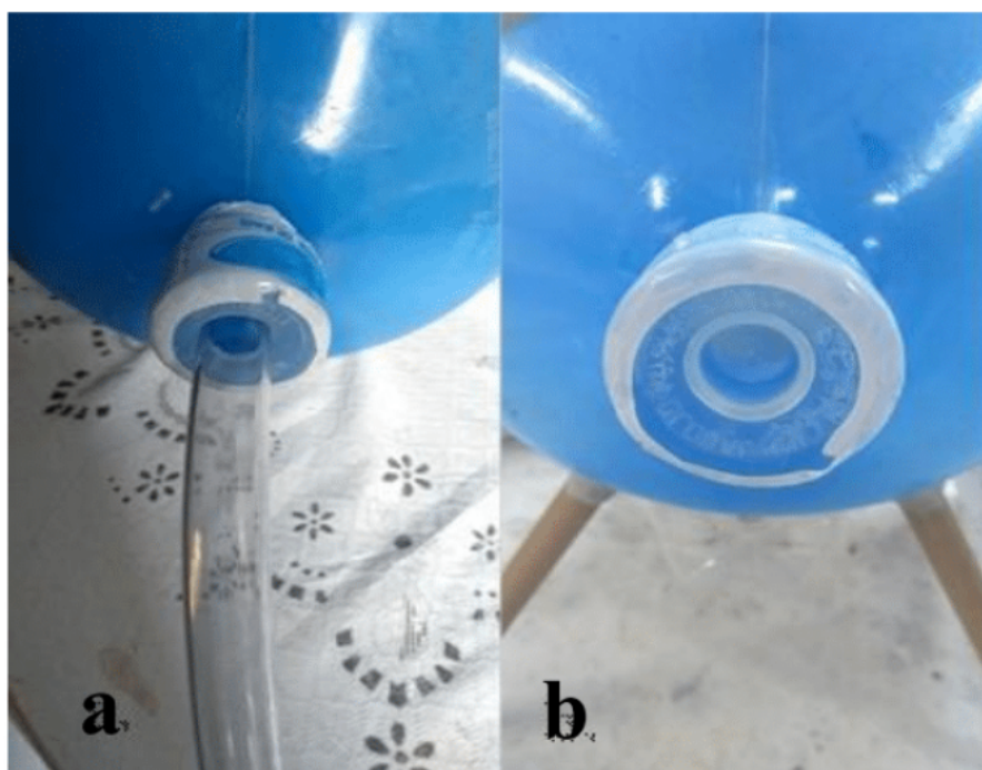
Figura 4. Local de abastecimento de água no destilador Autores (2019)
