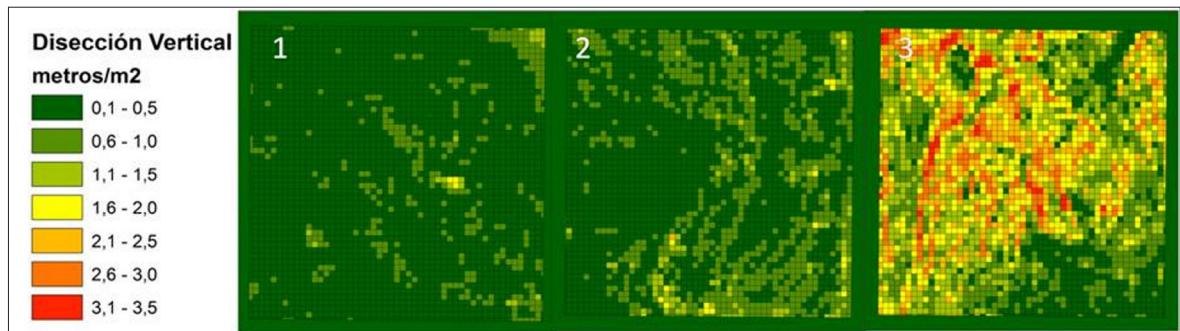
Figura 7. Mapa de disección vertical por litología: andesita (1), toba (2) y arcillas (3). Fuente: elaboración propia.
