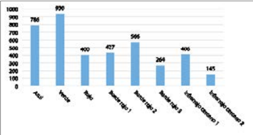
Figura 5. Número total de diferencias significativas encontradas por banda de Sentinel 2A. Fuente: elaboración propia.
