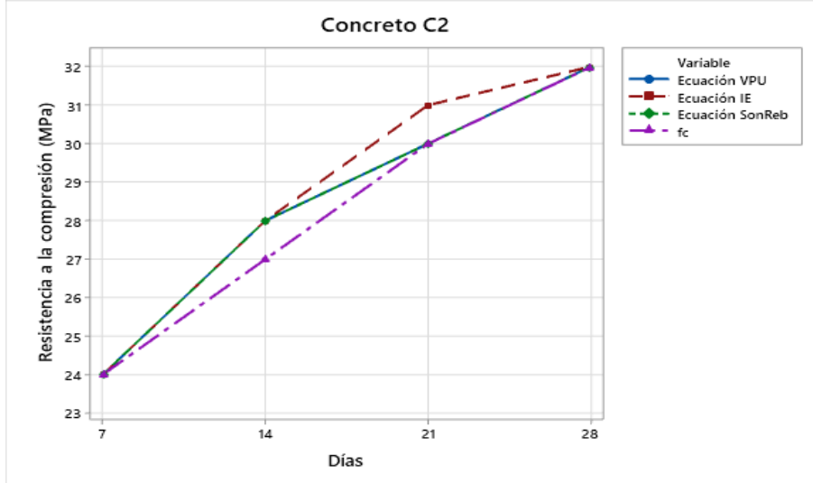
Figura 12. Análisis de la f'c mediante modelos de ecuaciones para concreto con adición de fibra de acero 5 %. Fuente: el autor
