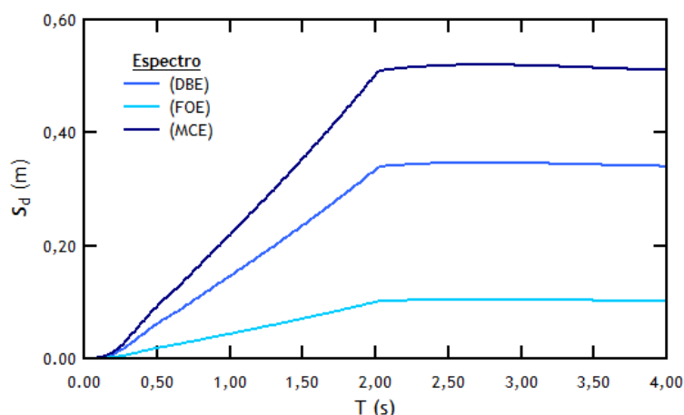
Figura 5. Espectros de aceleración para cada nivel de desempeño. Fuente: los autores
