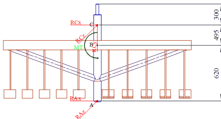
Figura 4. Diagrama de cuerpo libre del sistema
