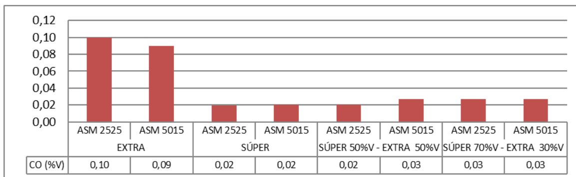
Figura 7. Cuadro comparativo del promedio de CO %Vol. en ASM 2525 y ASM 5015
