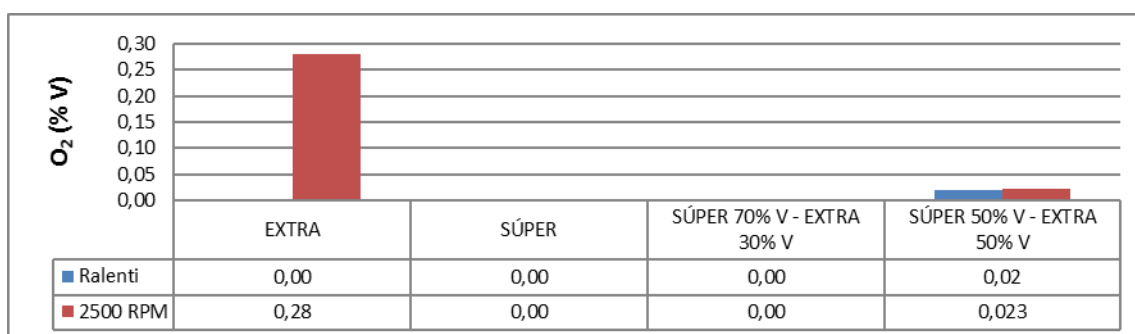
Figura 16. Comparación de valores de O 2 a ralenti y a 2500 rpm
