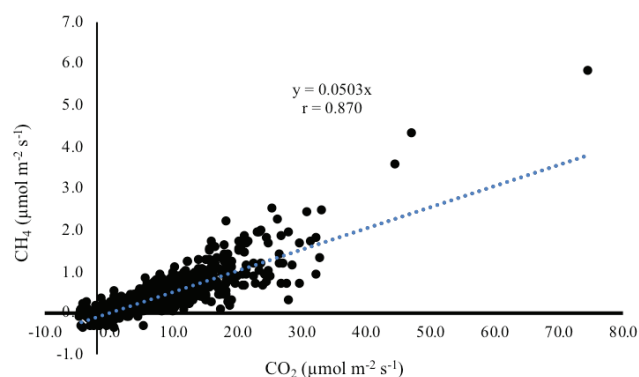
Figura 10. Razón de flujos de \text{CO}_2 y \text{CH}_4 en el corral con ganado lechero.
