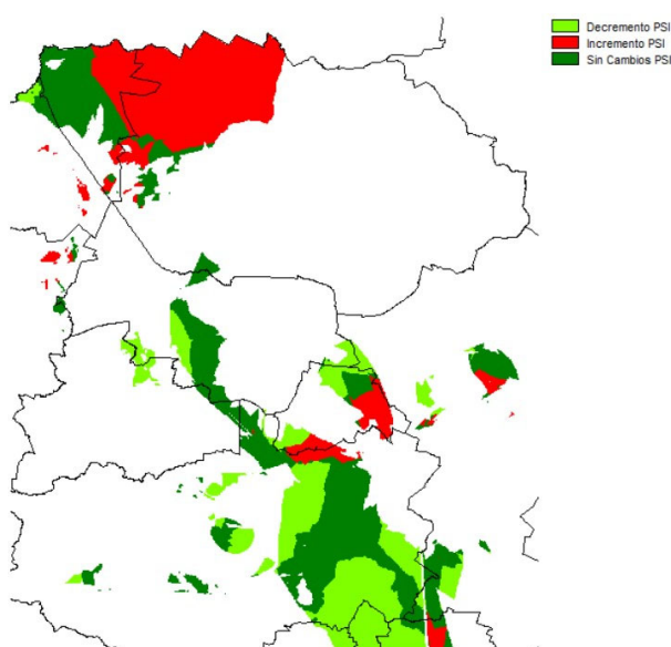
Figura 3. Cambios en valores de Porcentaje de Sodio Intercambiable de 1976 a 2016 en el norte de Zacatecas, México.
