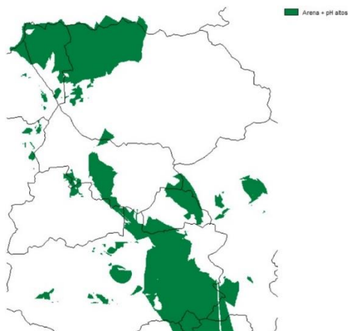
Figura 1. Área de coincidencia de acumulación de arena e incremento de valores de pH del suelo. Figure 1. Coincidence area of sand accumulation and increase in pH values.
