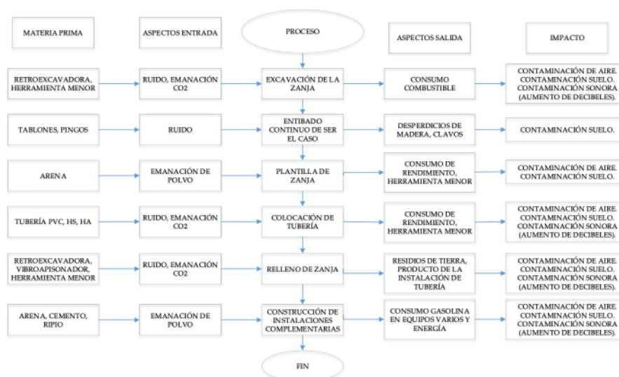
Figura 3 Modelo Eco-Mapa construcción de redes de alcantarillado con zanja Los Autores
