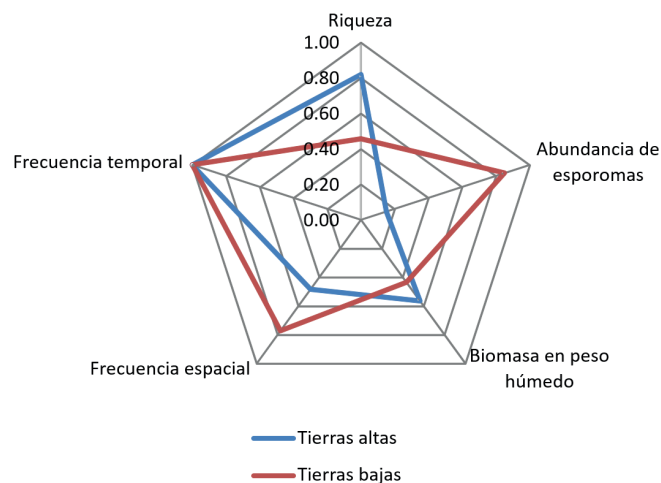
Figura 7: Disponibilidad multifactorial de esporomas de hongos silvestres en las tierras altas y bajas de Chiapas, México.
